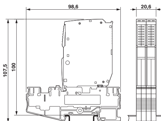
Maßzeichnung
