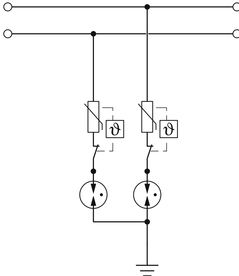
Anschlusszeichnung
