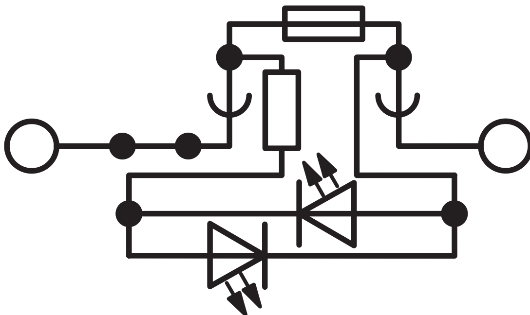
Schaltplan
