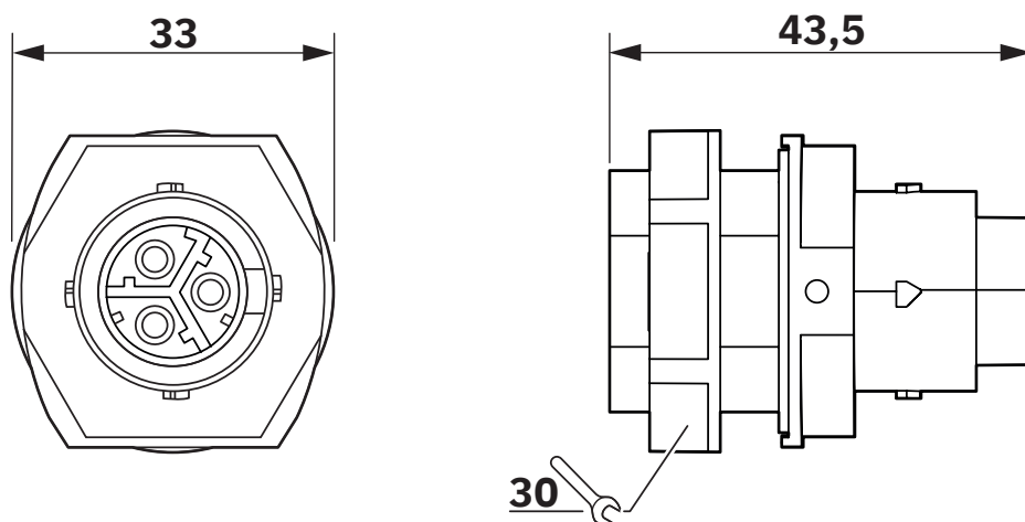
Maßzeichnung
