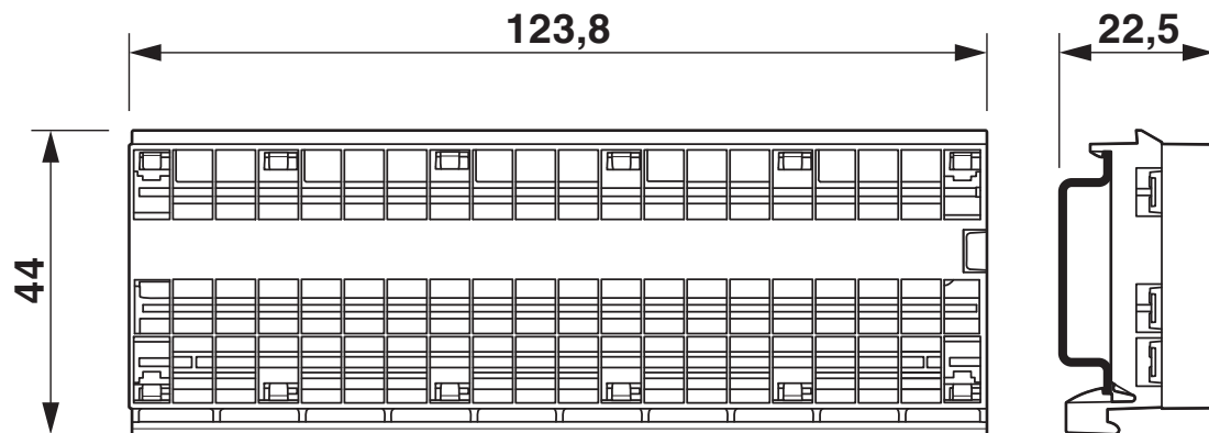
Maßzeichnung
