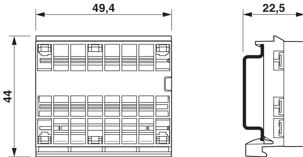
Maßzeichnung
