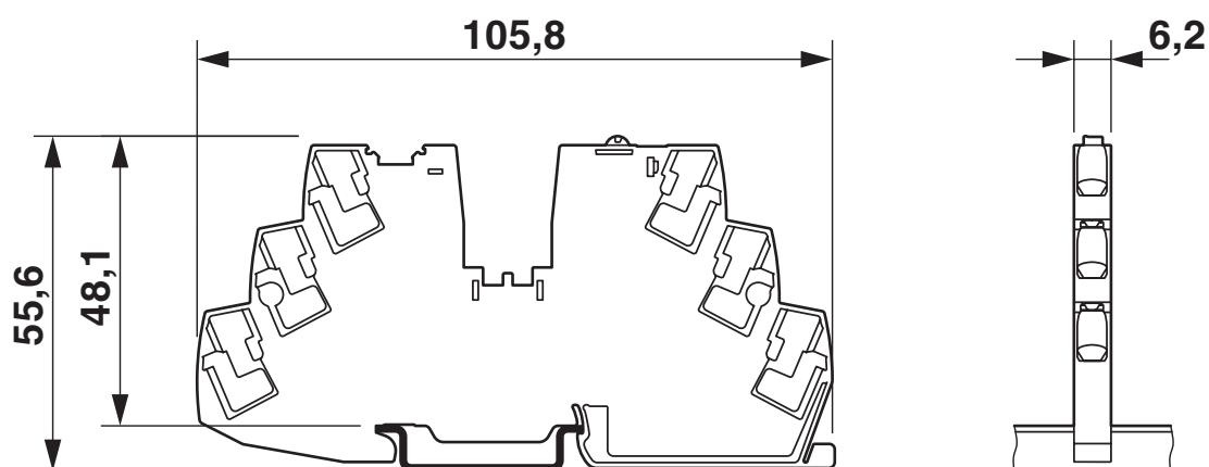
Maßzeichnung
