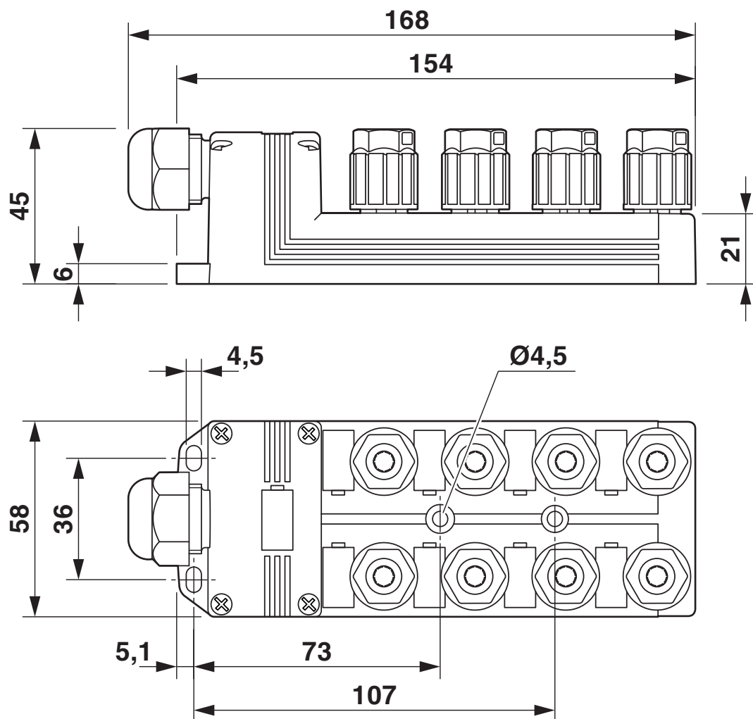
Maßzeichnung
