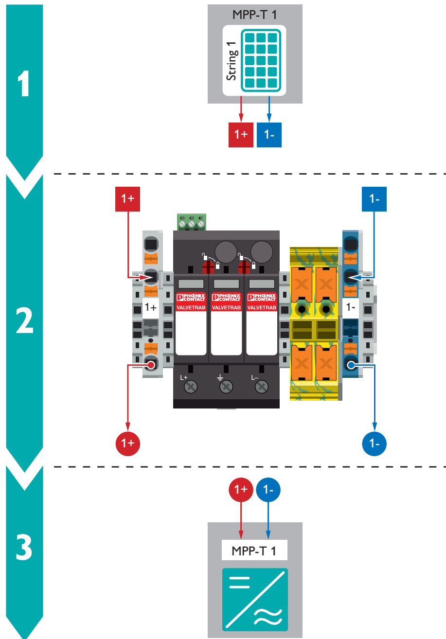
Schematische Applikationszeichnung
