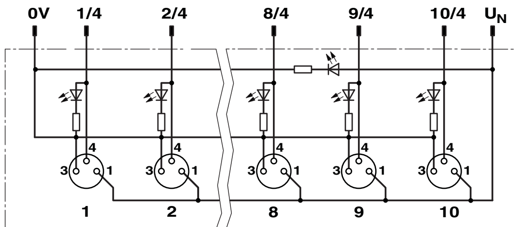
Schaltplan
