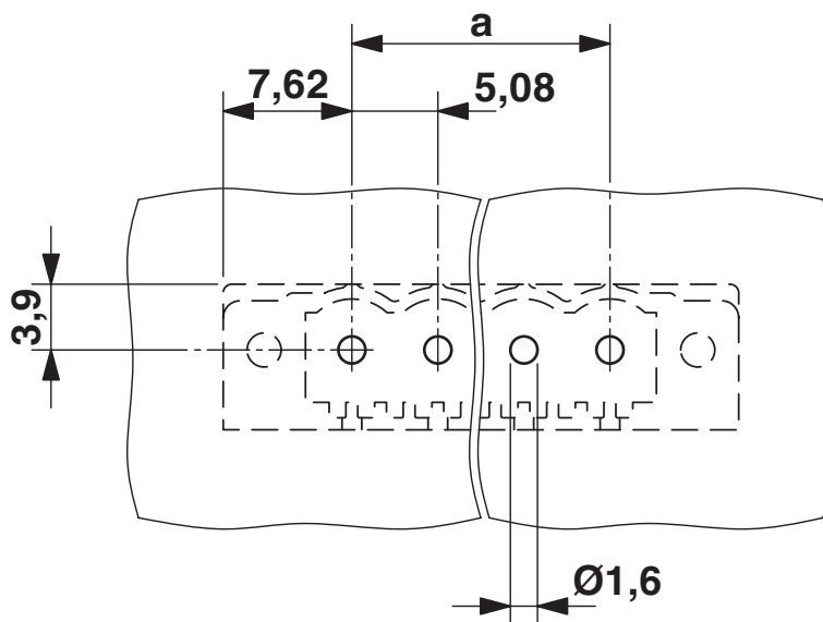
Bohrplan/Lötpadgeometrie
