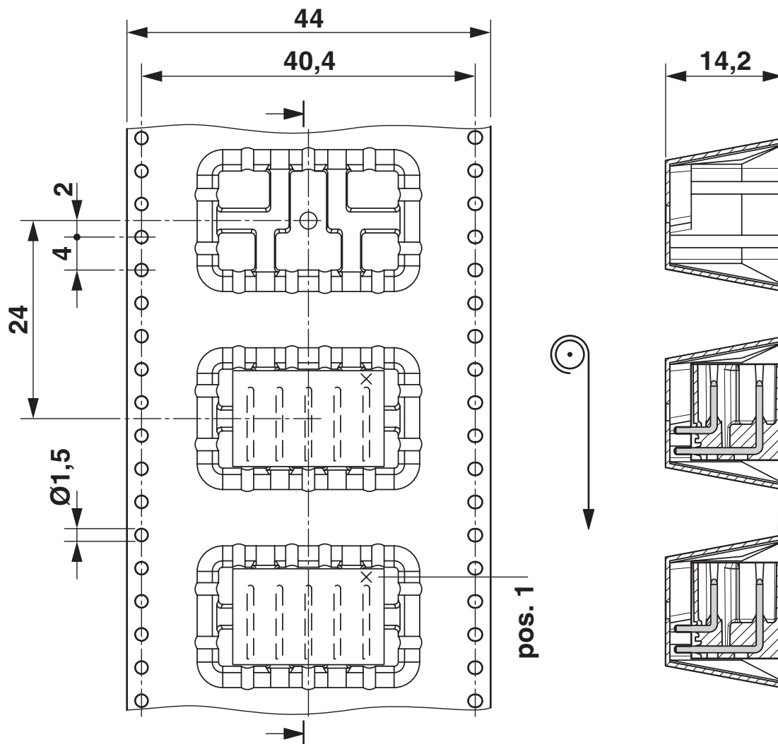
Maßzeichnung
