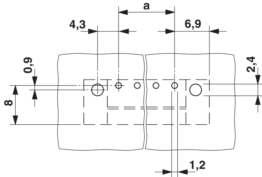
Bohrplan/Lötpadgeometrie
