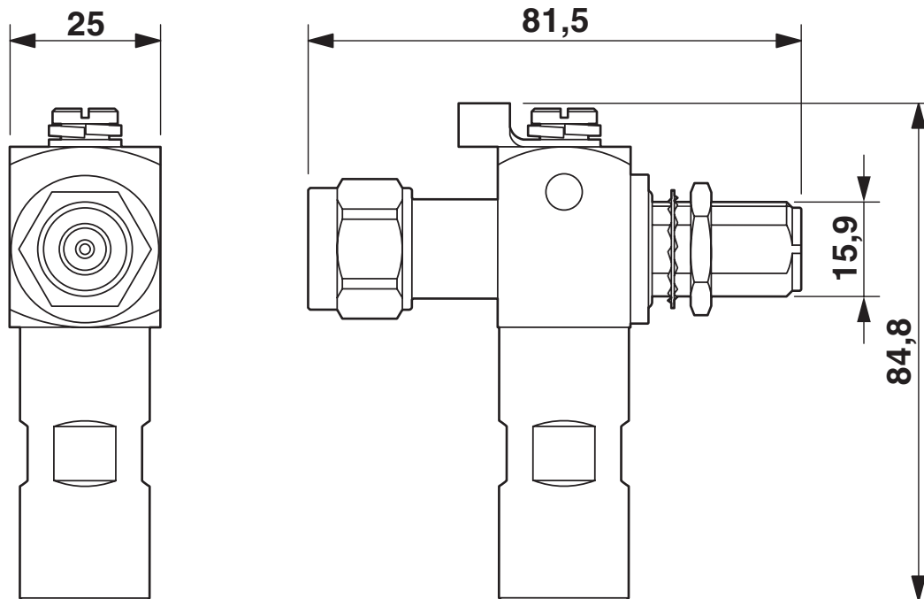
Maßzeichnung
