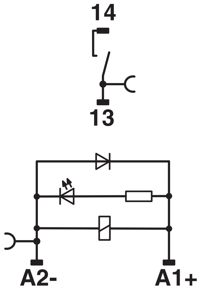
Schaltplan
