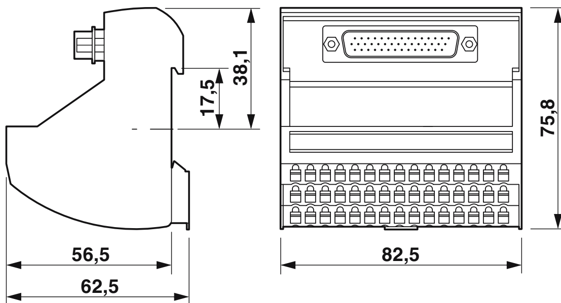
Maßzeichnung
