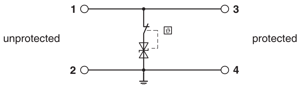
Schaltplan
