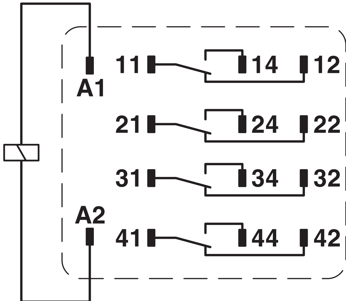
Schaltplan
