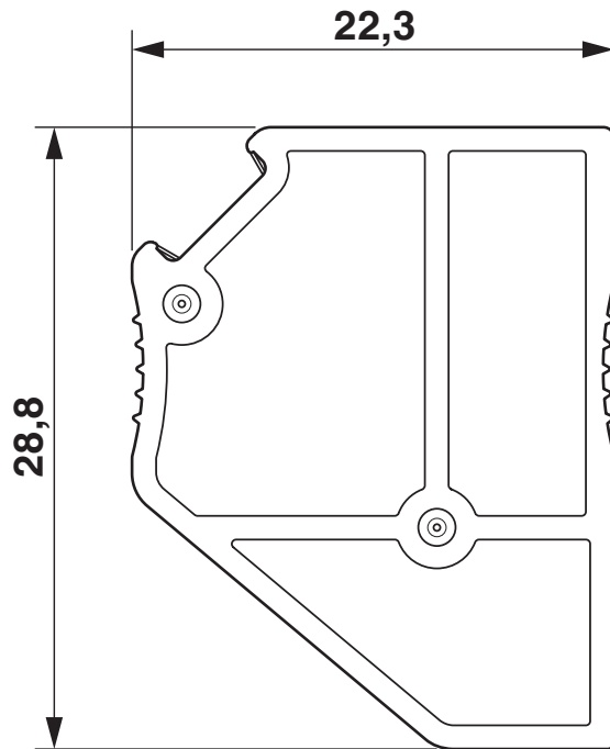
Maßzeichnung
