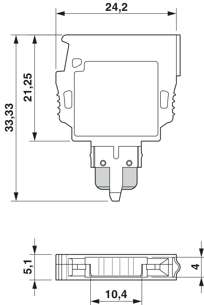
Maßzeichnung
