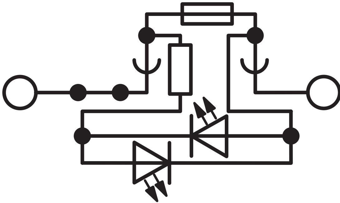
Schaltplan
