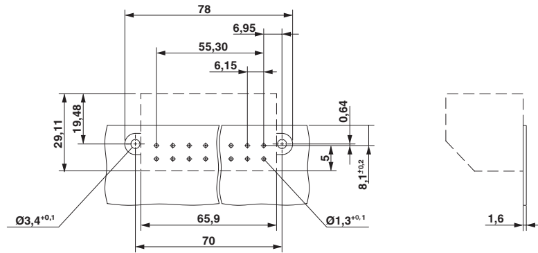
Maßzeichnung
