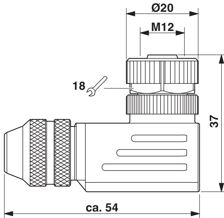
Maßzeichnung
