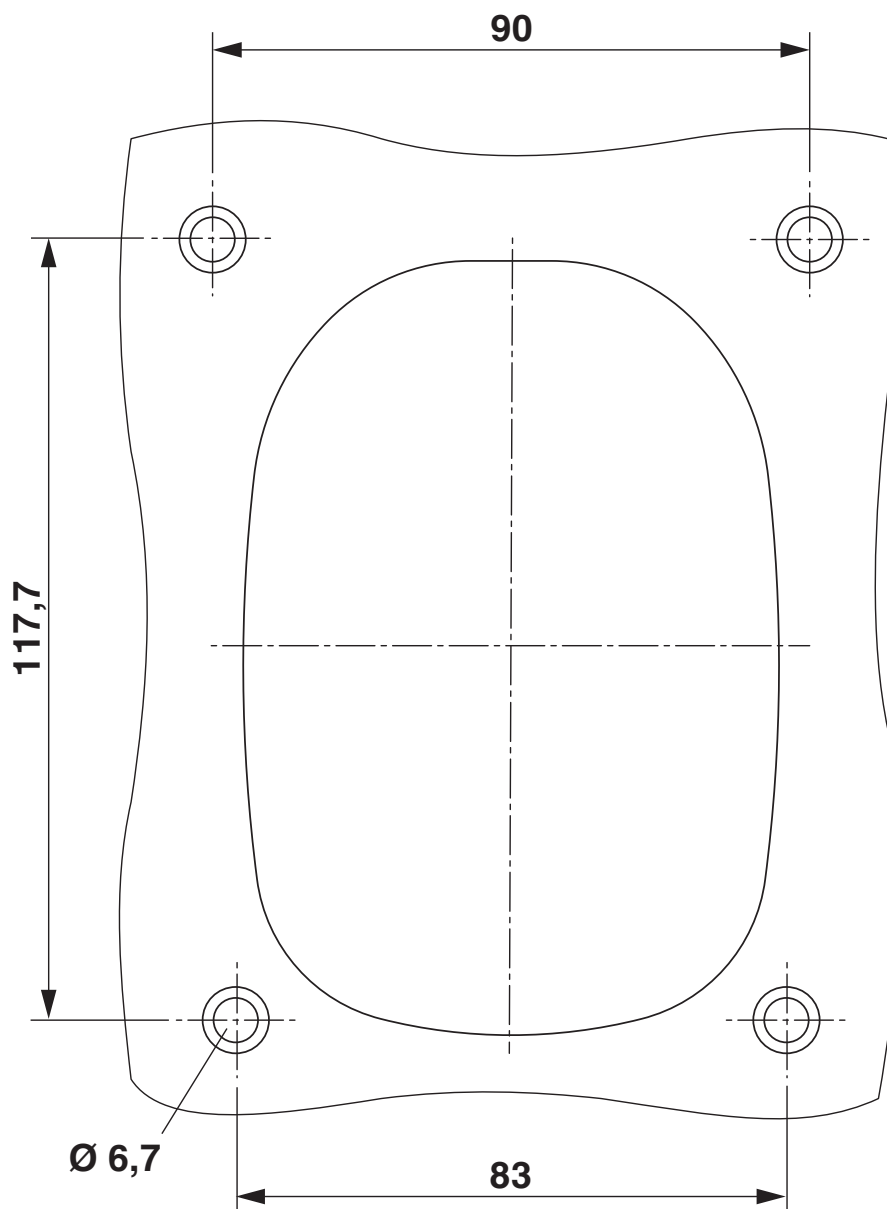
Bohrplan/Lötpadgeometrie
