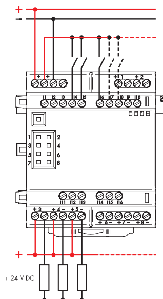
Typ 8A.88-160x
