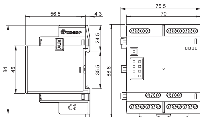
Typ 8A.26-060x Käfigklemmen
