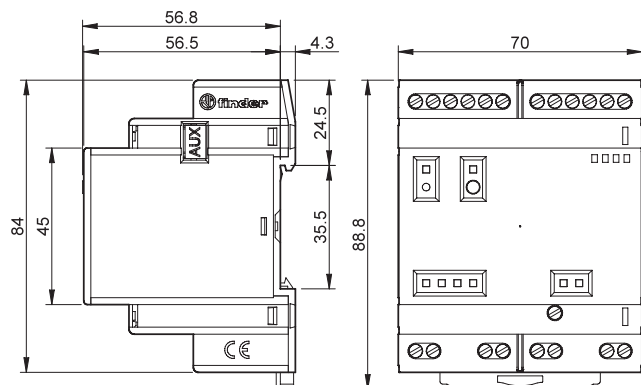
Typ 8A.58-160x Käfigklemmen
