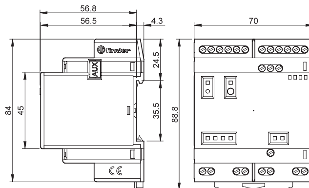
Typ 8A.88-160x Käfigklemmen
