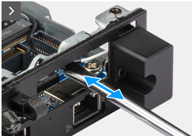
Abbildung 58. Installieren des Glasfasermoduls
