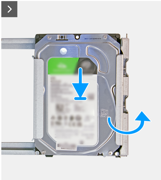
Abbildung 22. Einsetzen des Festplattenlaufwerks
