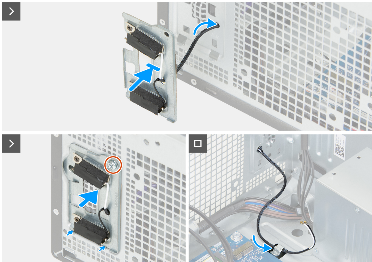
Abbildung 32. Einbauen des Antennenmoduls
