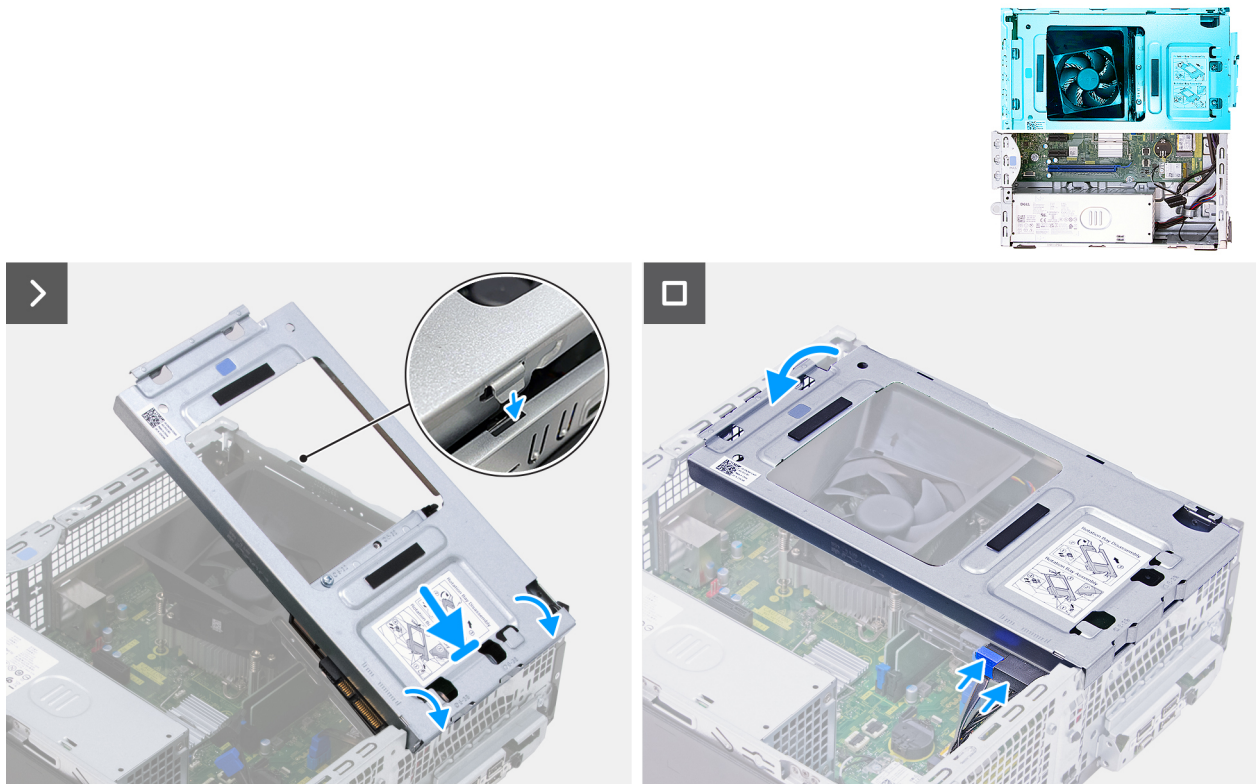
Abbildung 20. Einbauen des Laufwerkschachts
