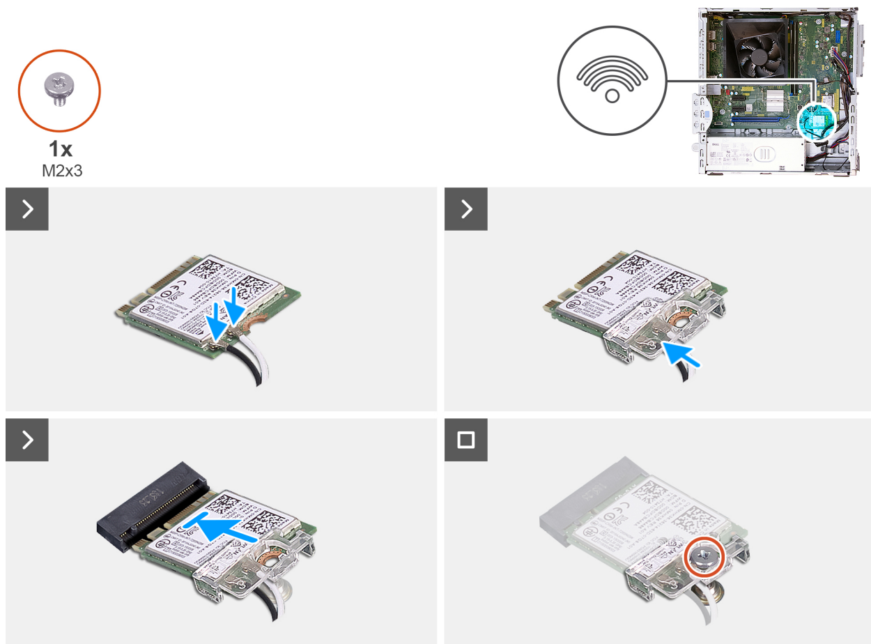
Abbildung 28. Installieren der Wireless-Karte
