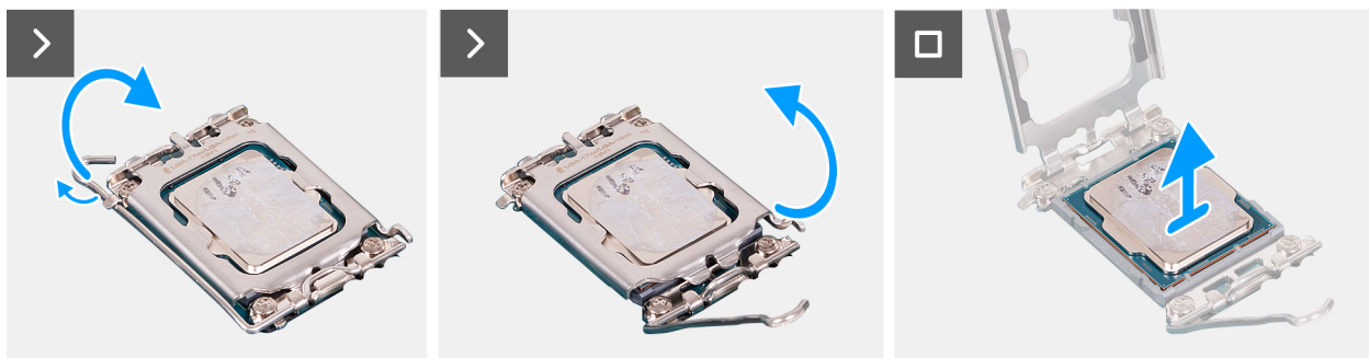
Abbildung 41. Entfernen des Prozessors
