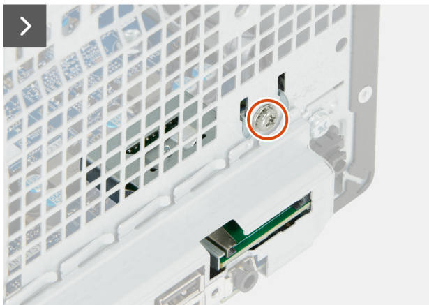
Abbildung 29. Entfernen des Medienkartenlesegeräts
