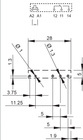
Ansicht auf die Anschlüsse
