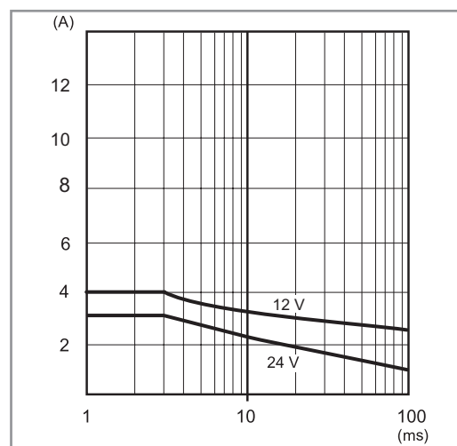
P78-3 Einschaltspitzenstrom-Belastbarkeit (78.25)
