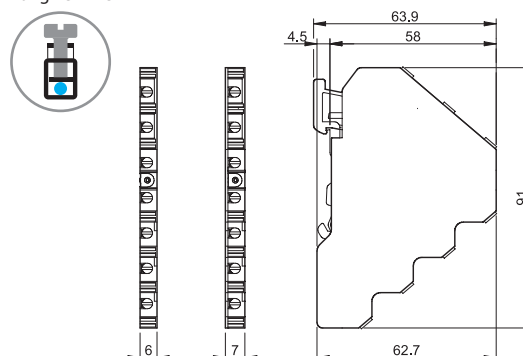
Typ 7P.62.9.036.0005/7P.62.9.009.0485 Käfigklemmen
