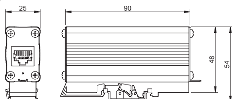
Typ 7P.68.9.060.0600 RJ45-Buchse
