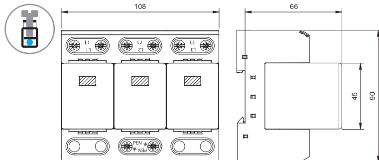
Typ 7P.03 Käfigklemmen
