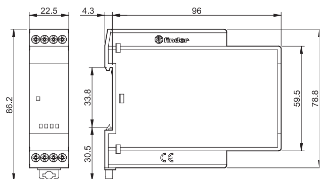
Typ 75.36 Käfigklemmen
