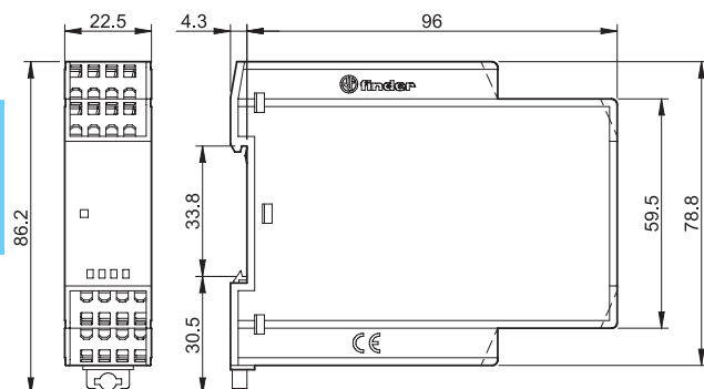
Typ 75.32 Käfigklemmen
