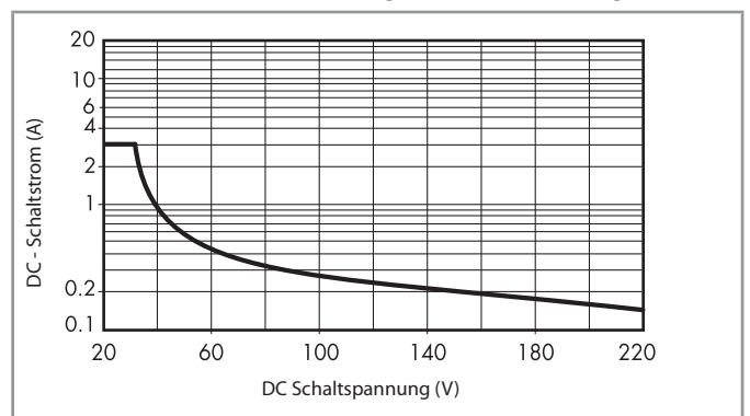
H 7S16/36 - Gleichstromschaltvermögen bei DC13-Belastung - 7S.16/36
