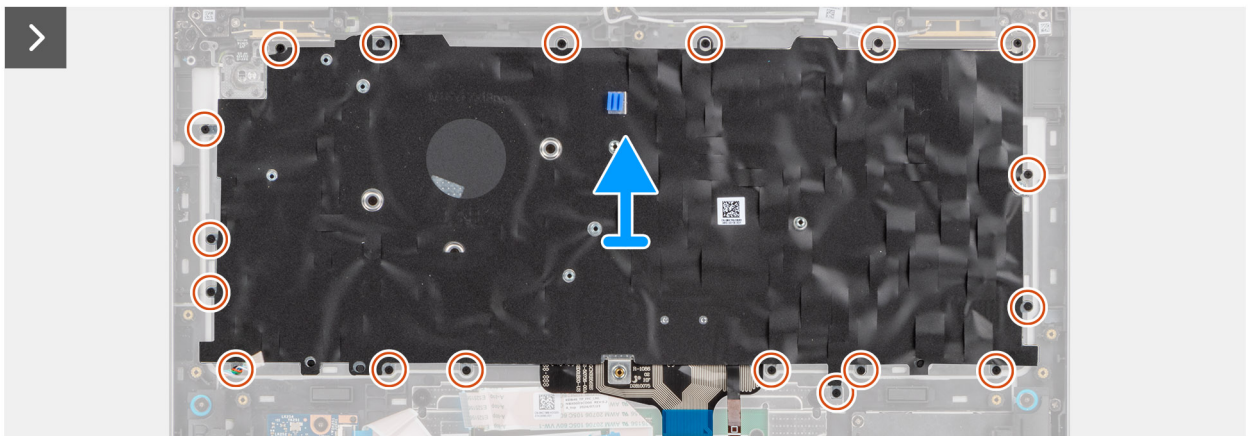
Abbildung 81. Entfernen der Tastatur
