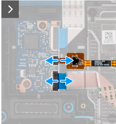
Abbildung 43. Entfernen der USH-Platine
