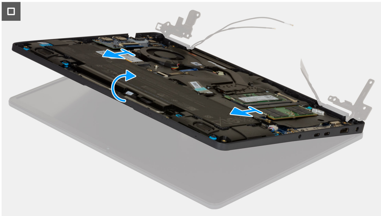
Abbildung 100. Entfernen der Bildschirmbaugruppe
