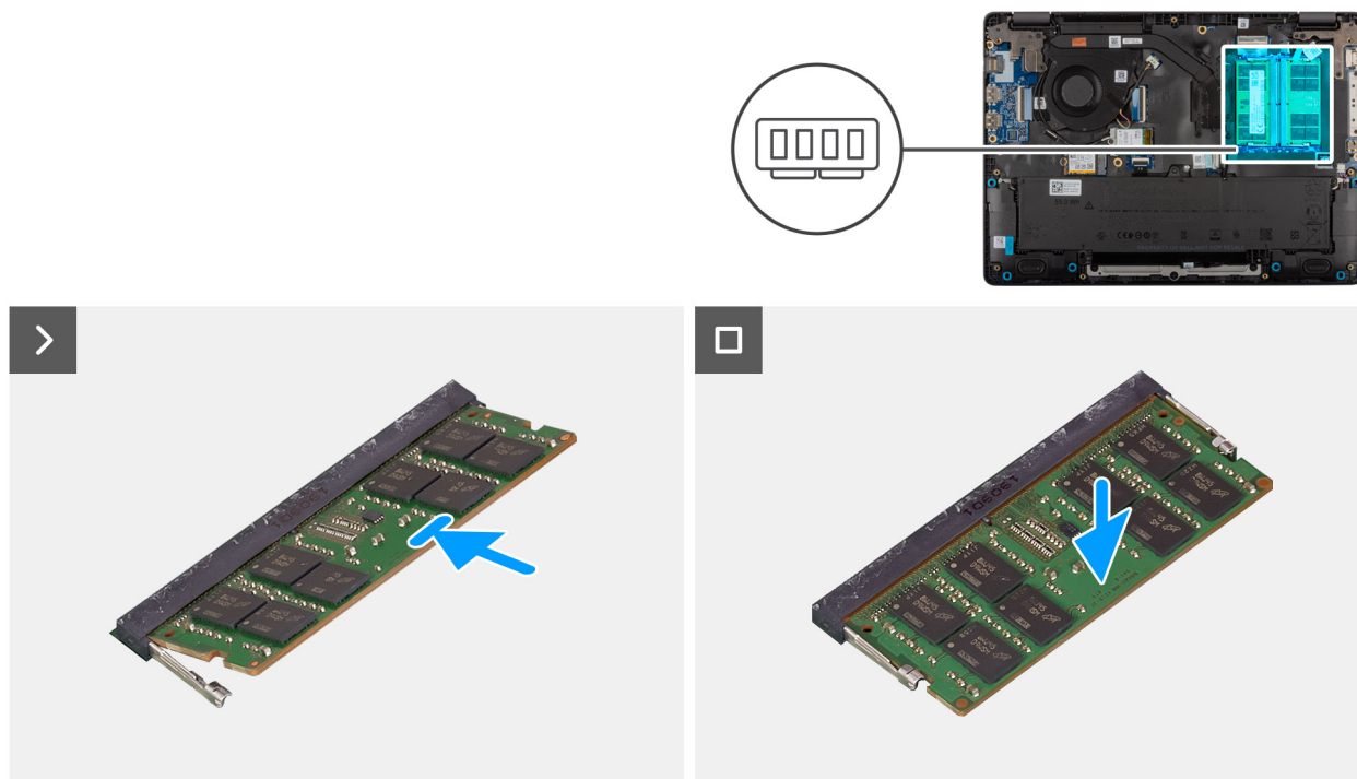
Abbildung 22. Installieren der Speichermodule
