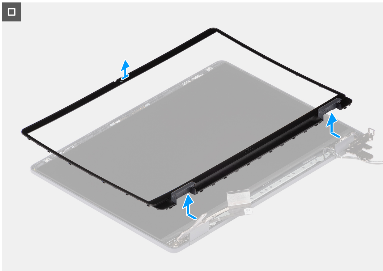
Abbildung 108. Entfernen der Bilderamblende
