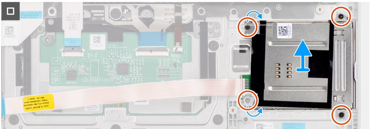
Abbildung 39. Entfernen des Smartcardlesegeräts
