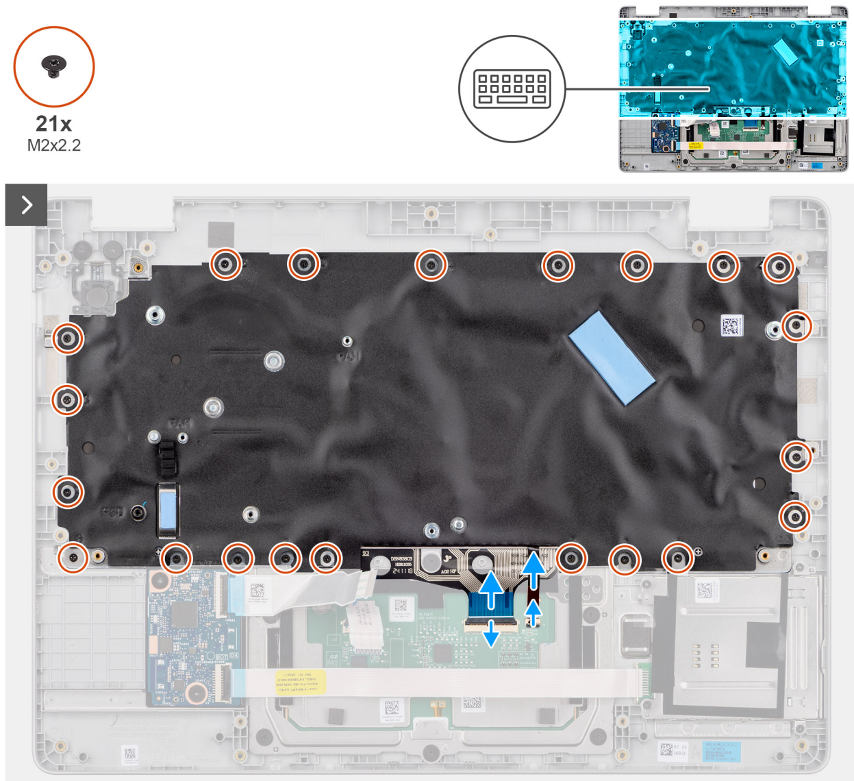
Abbildung 85. Entfernen der Tastatur
