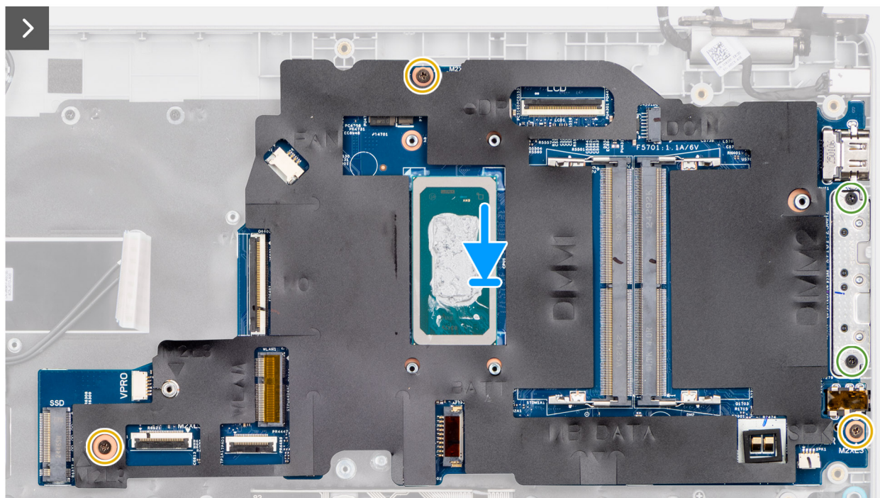
Abbildung 73. Einbauen der Systemplatine
