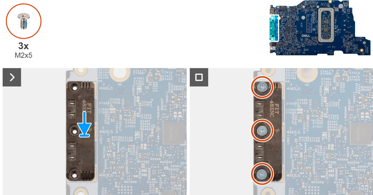
Abbildung 76. Installieren des USB-Typ-C-Moduls
