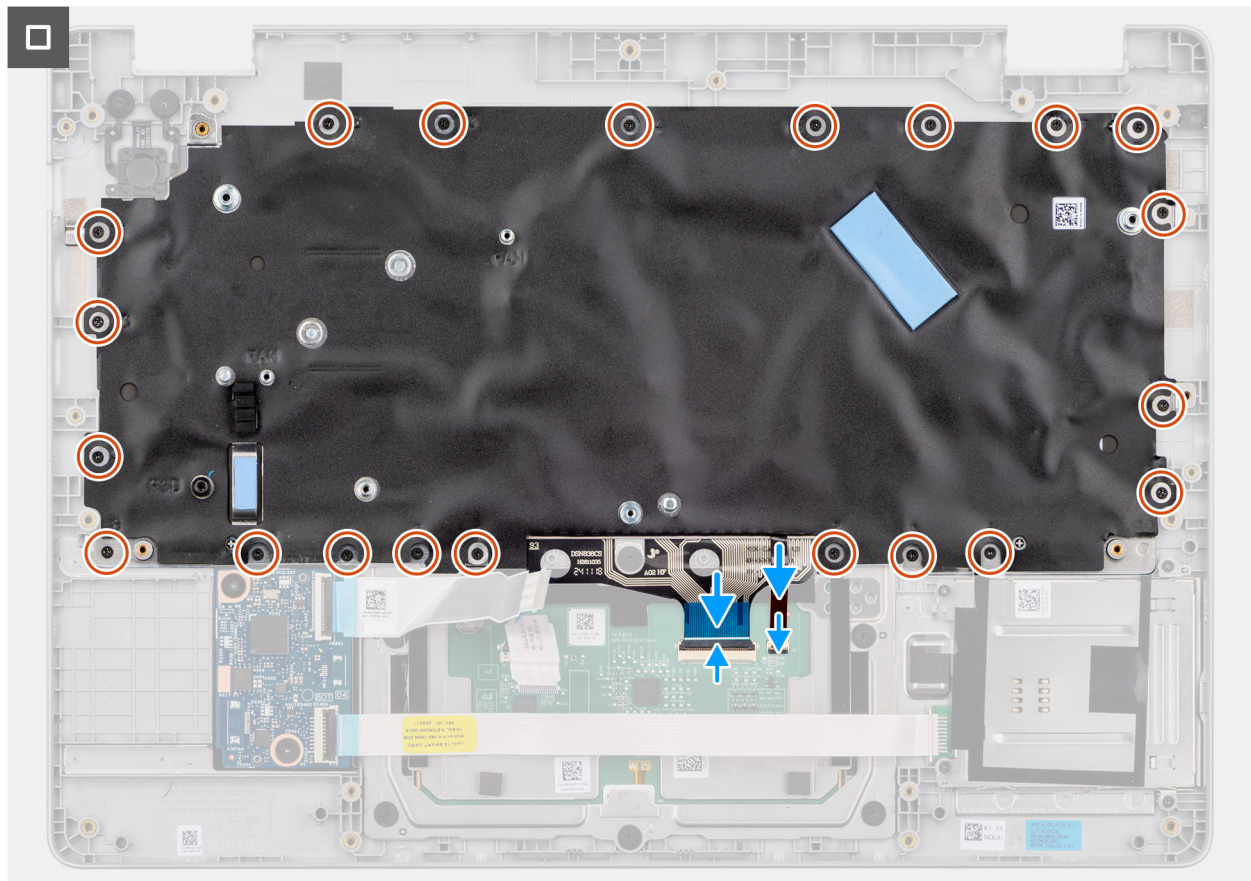
Abbildung 90. Einbauen der Tastatur
