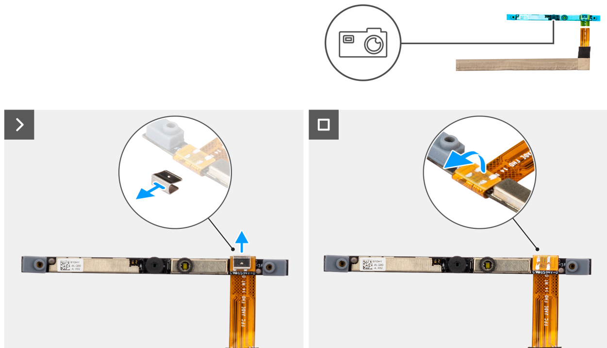
Abbildung 119. Entfernen der Kamera
