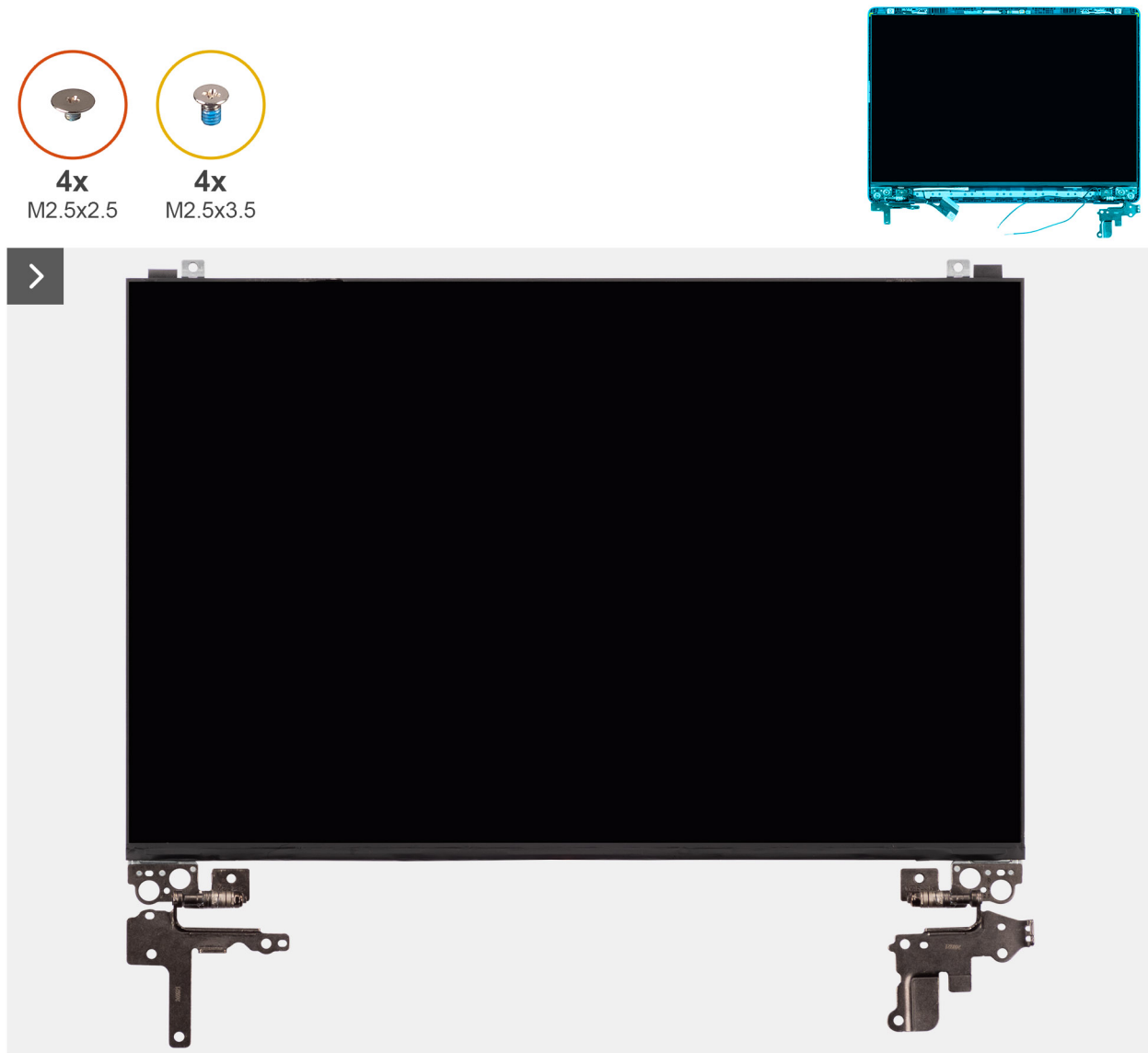
Abbildung 115. Installieren der Bildschirmbaugruppe
