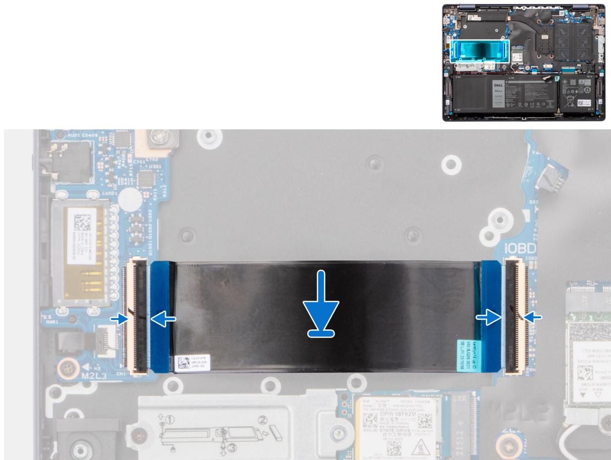
Abbildung 42. Installieren des I/O-Platinkabels
