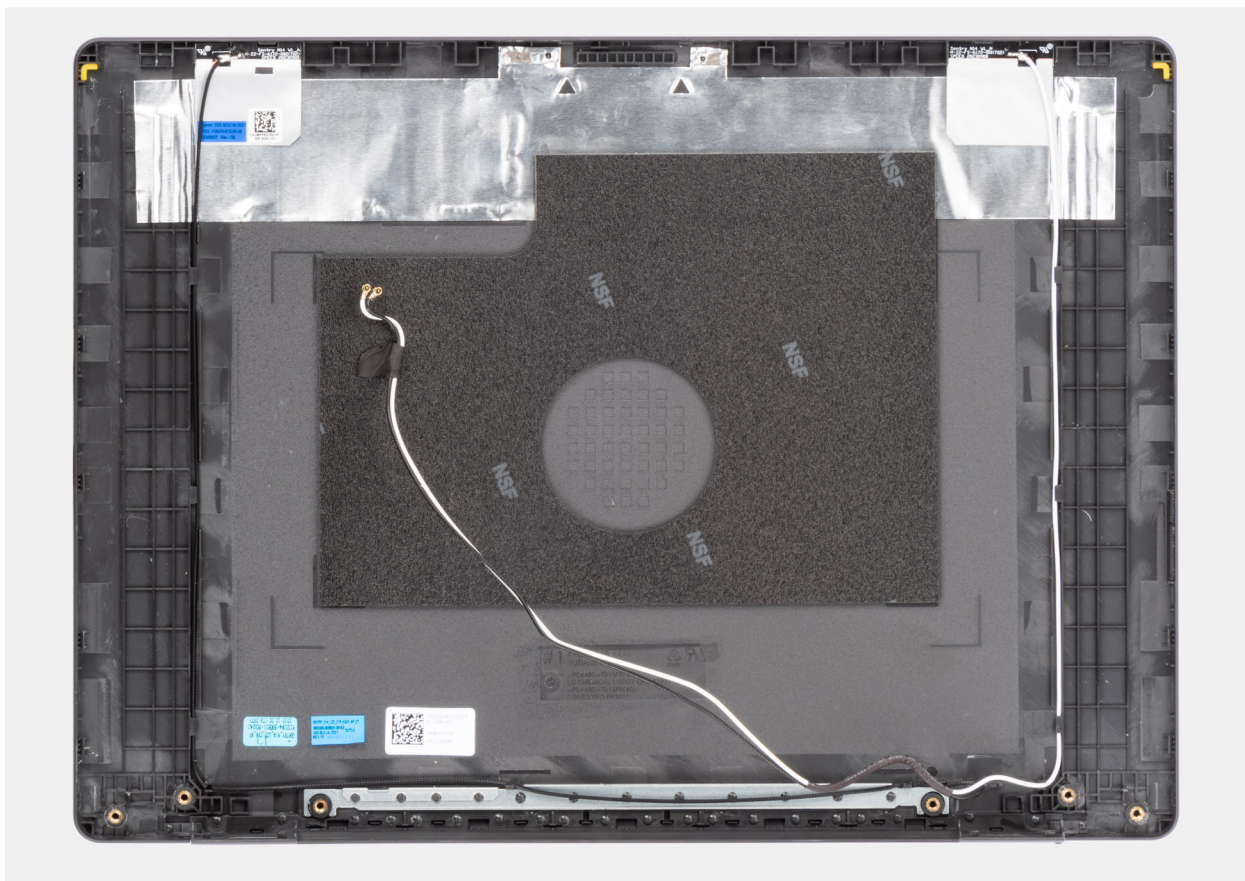
Abbildung 77. Bildschirmrückwand-Antennen-Baugruppe
