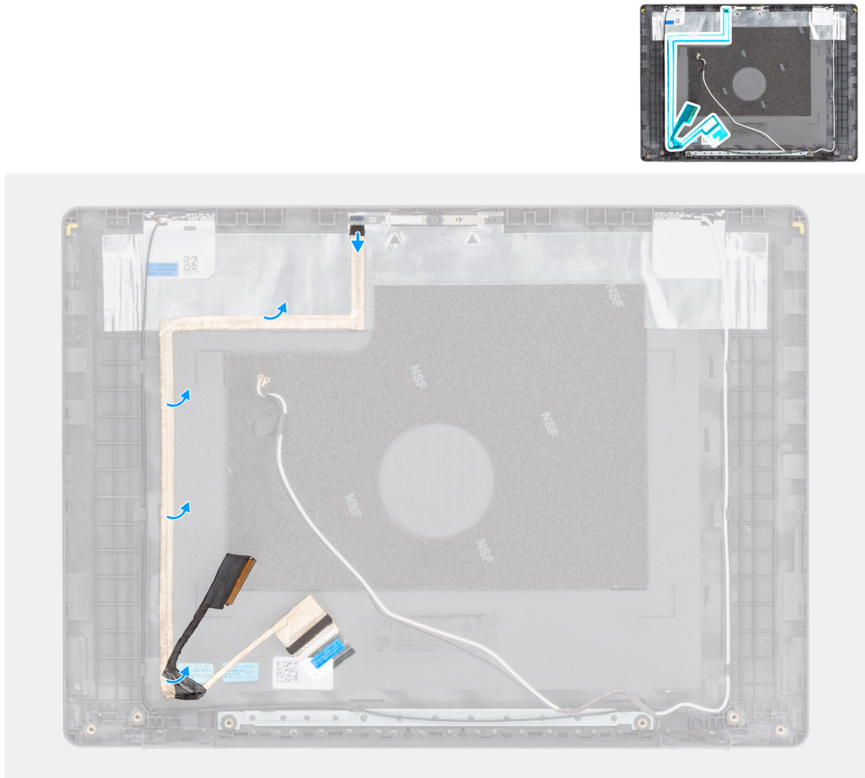
Abbildung 72. Entfernen des Bildschirmkabels
