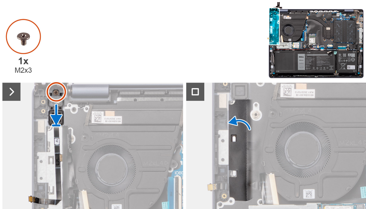
Abbildung 50. Einbauen des Netzschalters mit optionalem Fingerabdruckleser
