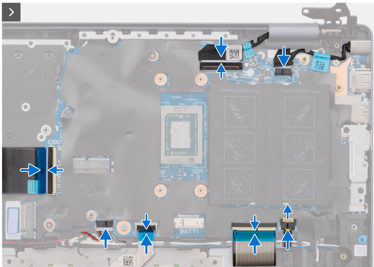
Abbildung 94. Einbauen der Systemplatine (bei Computern mit Aluminiumgehäuse)
