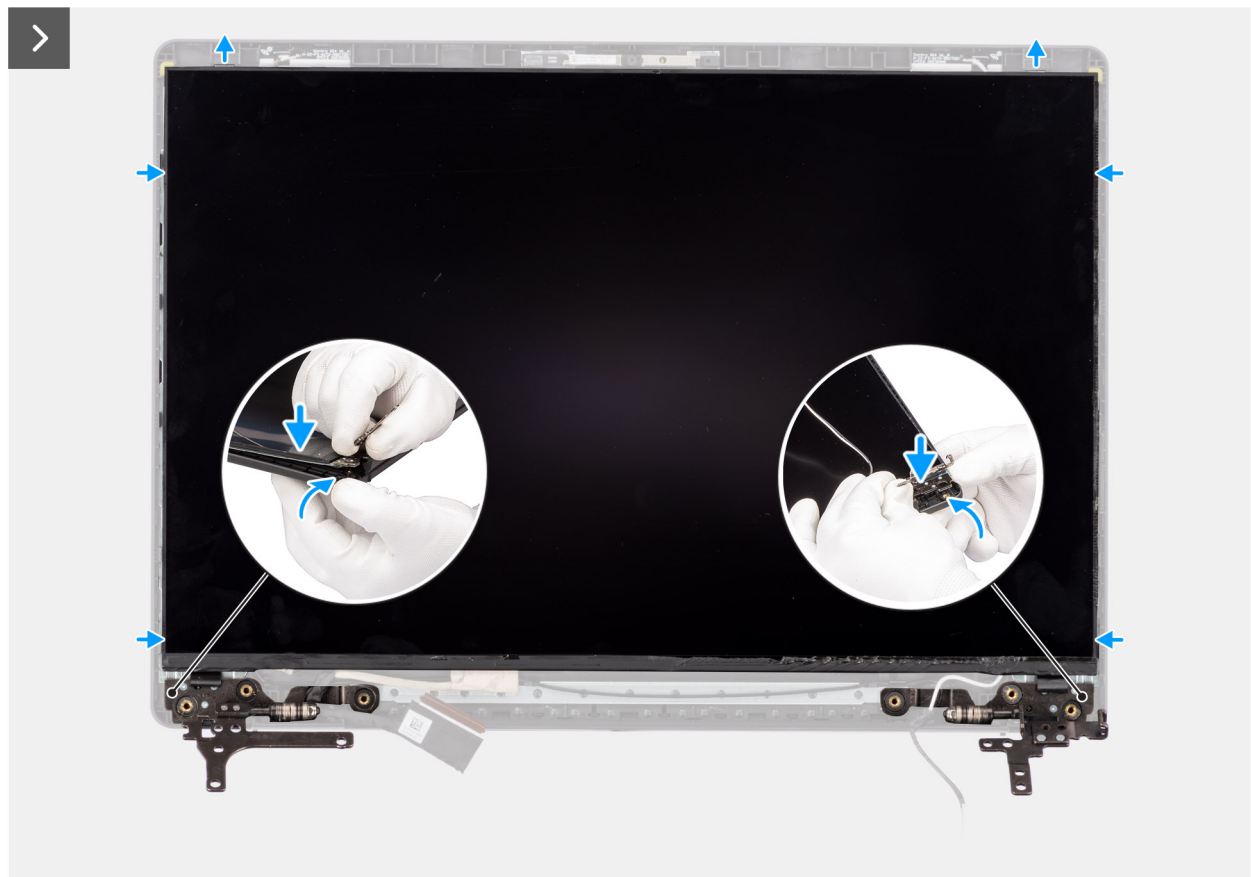
Abbildung 70. Installieren des Bildschirms
