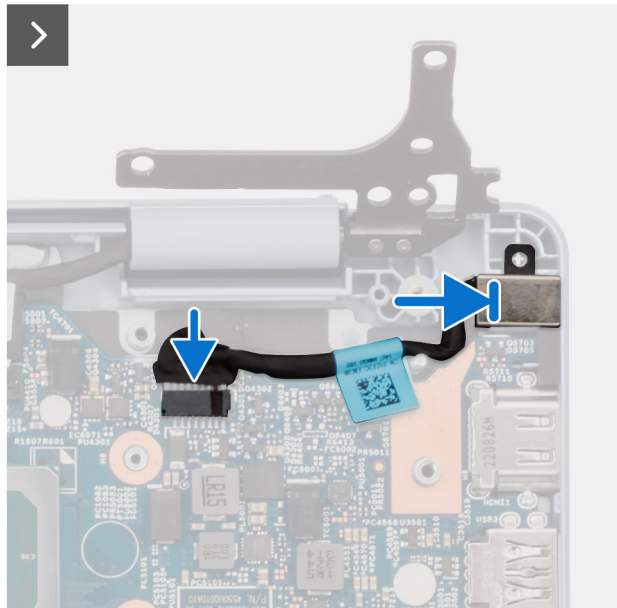
Abbildung 47. Einbauen des Netzadapter-Ports
