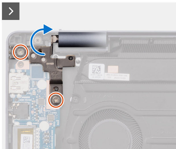
Abbildung 70. Entfernen der Schrauben
