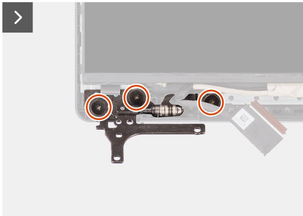
Abbildung 76. Entfernen der Bildschirmschrauben
