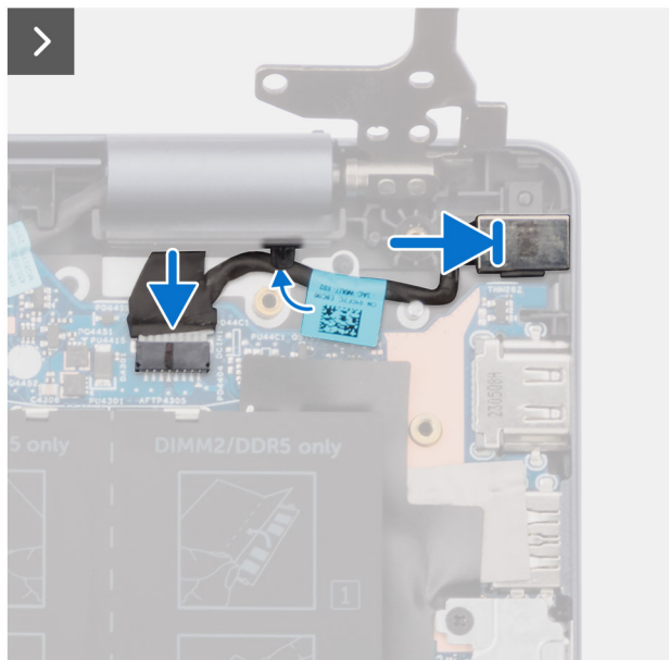
Abbildung 49. Einbauen des Netzadapter-Ports
