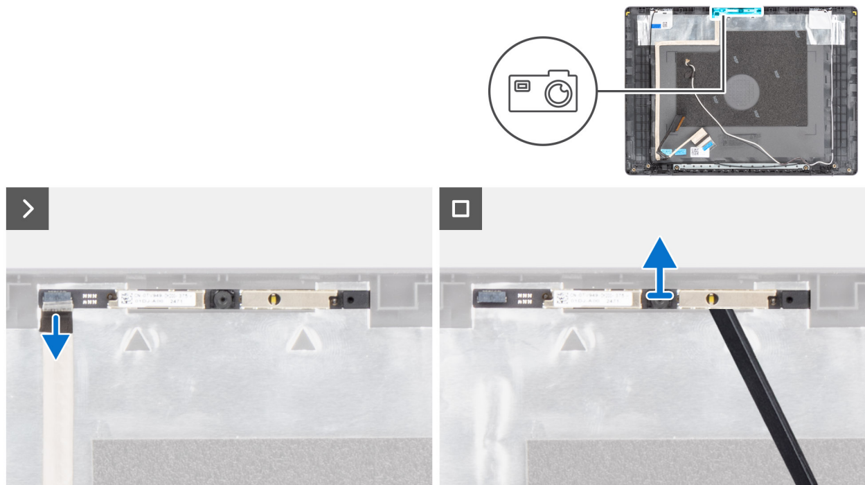
Abbildung 87. Entfernen der Kamera
