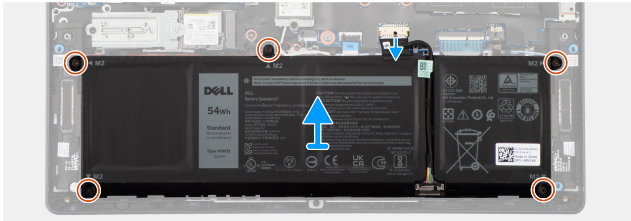
Abbildung 24. Entfernen des Akkus
