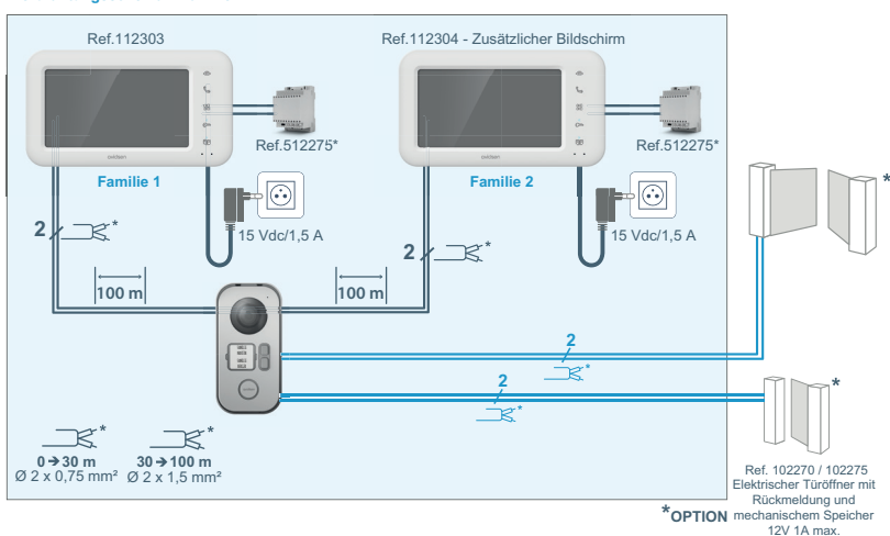
Verdrahtungsschema 2 Familien
