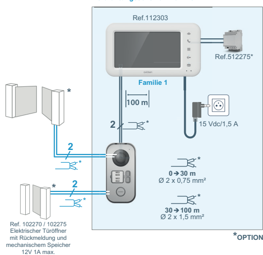
Verdrahtungsschema 1 Familie
