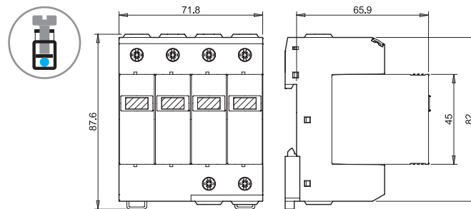
Typ 7P.15 Käfigklemmen
