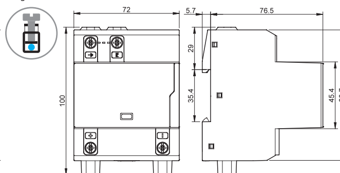
Typ 7P.13.9.500.x006 Käfigklemmen
