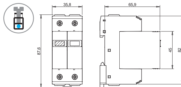
Typ 7P.22/7P.27/7P.42 Käfigklemmen
