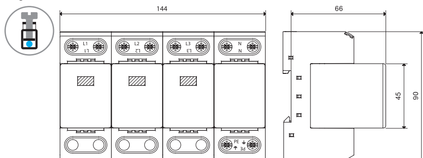
Typ 7P.04 Käfigklemmen
