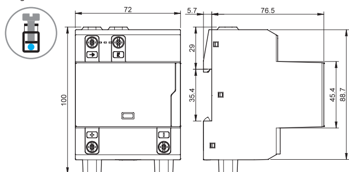
Typ 7P.13.9.000.x006 Käfigklemmen
