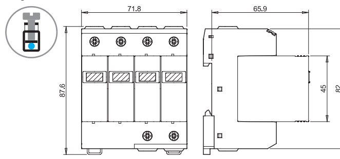
Typ 7P.25/7P.45 Käfigklemmen
