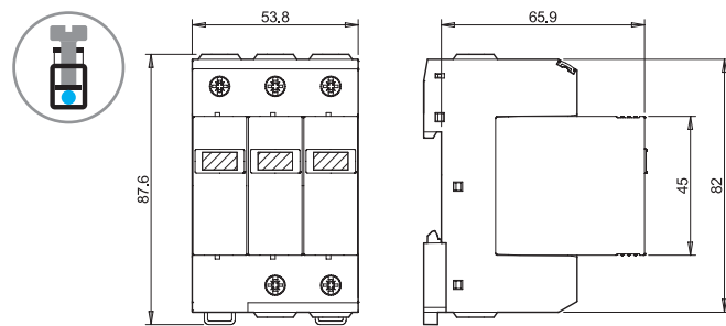
Typ 7P.13 Käfigklemmen
