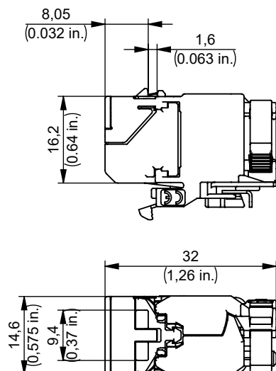
Einbaumaße / mounting dimensions
