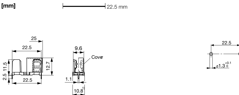
Bohrplan
