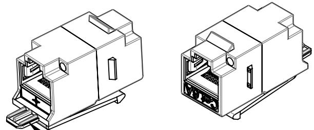
Flachstecker 6,3 mm DIN46342-1 für Funktionserdung IEC60364-5-54 blade terminal 6,3 mm DIN46342-1 for functional earthing acc. to IEC60364-5-54
