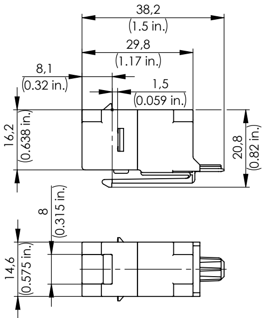
Einbaumaße (max. und min.) mounting dimension (max. and min.)
