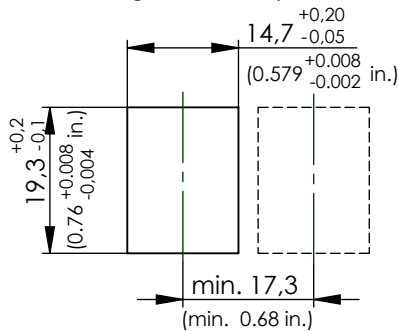
Materialdicke 1,5 \pm 0,05 mm wall thickness 1,5 \pm 0,05 mm (0.059 \pm 0.002 in.)
