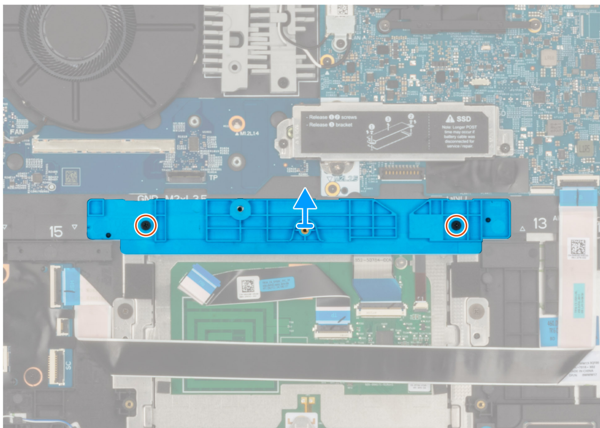
Abbildung 39. Akkuhalterung
