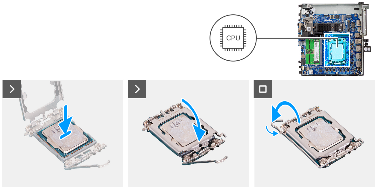
Abbildung 50. Einbauen des Prozessors
