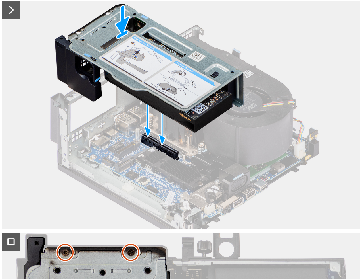
Abbildung 11. Einbauen des Riser-Kartenmoduls
