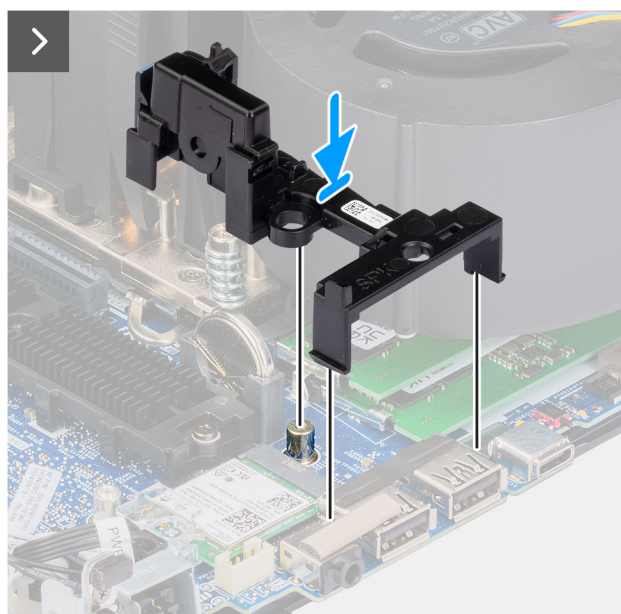
Abbildung 31. Einbauen der Lautsprecherbauhalterung
