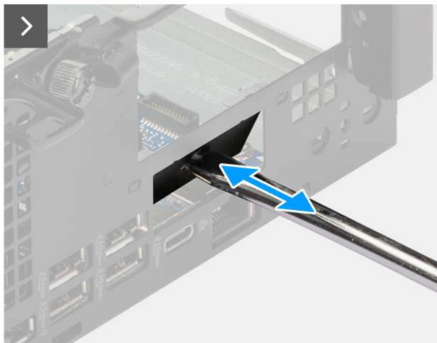
Abbildung 35. Einbauen des PS2-Anschlusses
