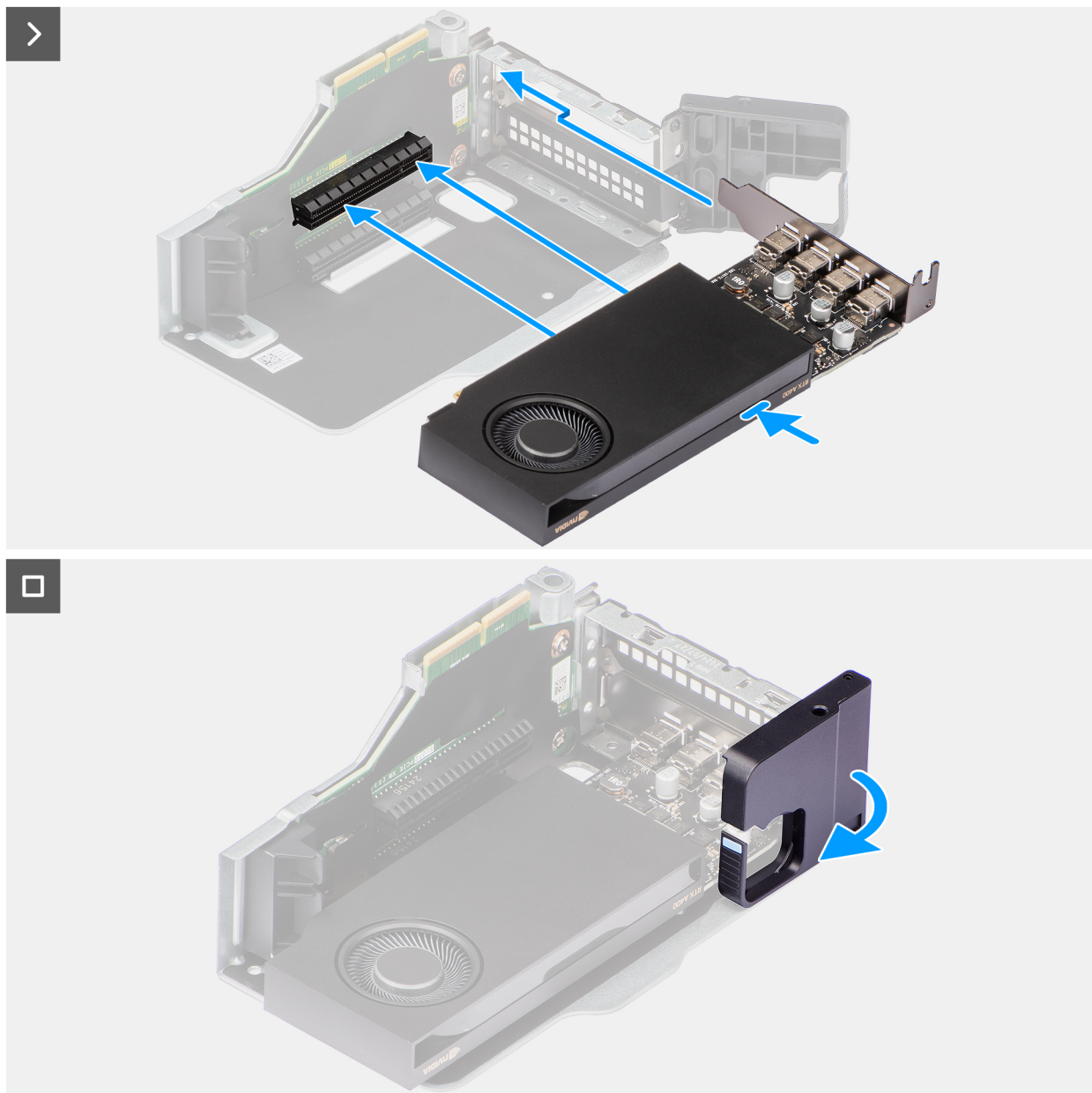
Abbildung 15. Installieren der Grafikkarte
