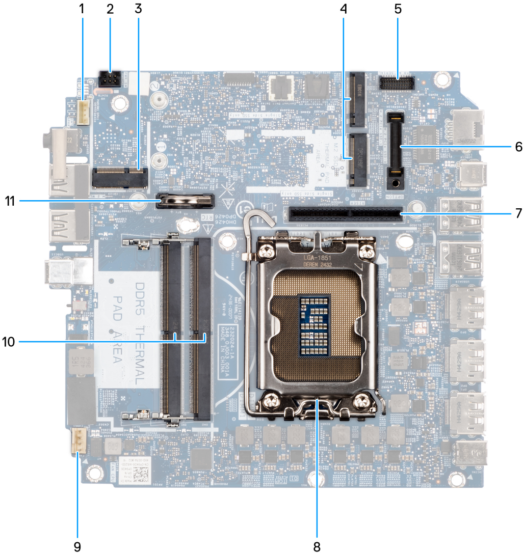
Abbildung 51. Anschlüsse auf der Hauptplatine
