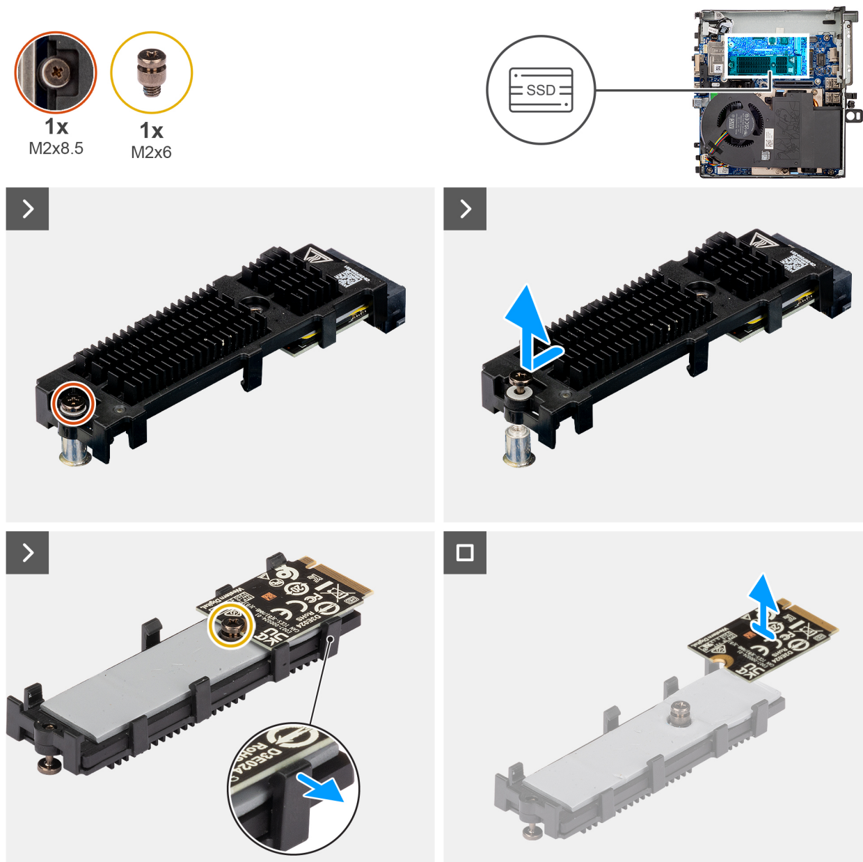
Abbildung 20. Entfernen des M.2-2230-PCIe-Solid-State-Laufwerks (Steckplatz 1)
