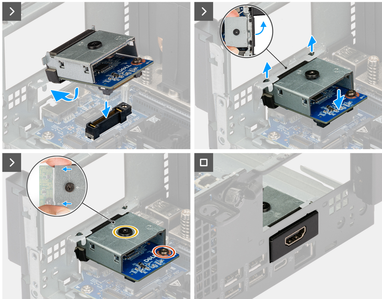
Abbildung 45. Einbauen des HDMI-Ports
