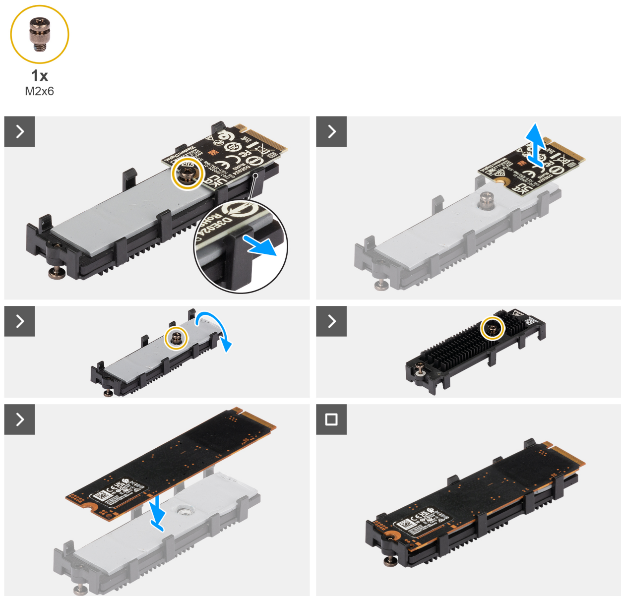
Abbildung 24. Ersetzen der M.2-2230-SSD durch eine M.2-2280-SSD
