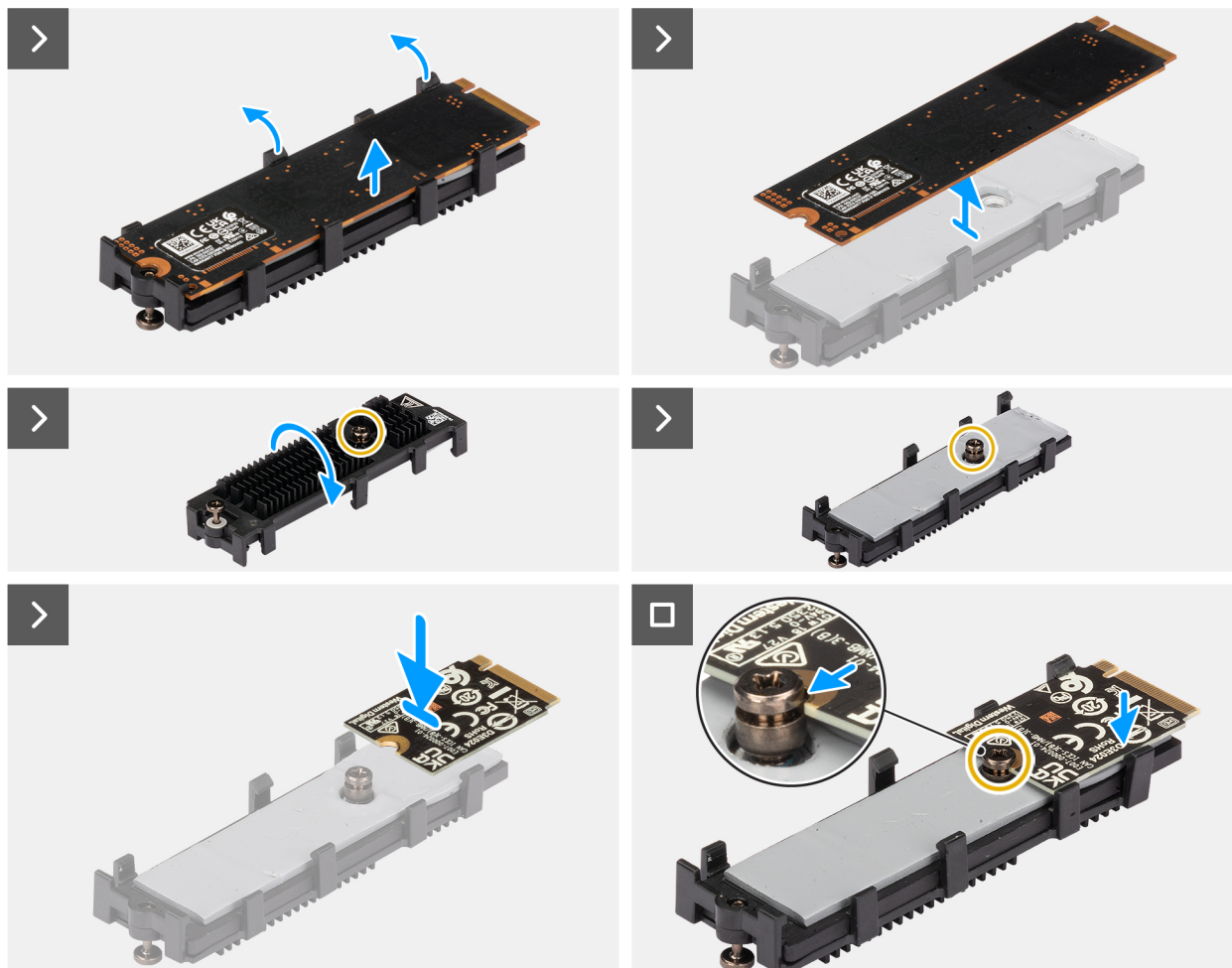
Abbildung 25. Ersetzen der M.2-2280-SSD durch eine M.2-2230-SSD
