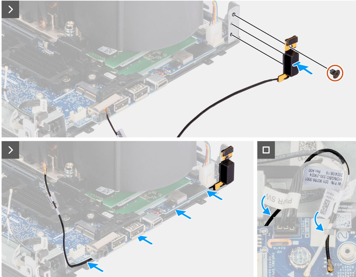
Abbildung 62. Einbauen der internen Antenne – Position 2
