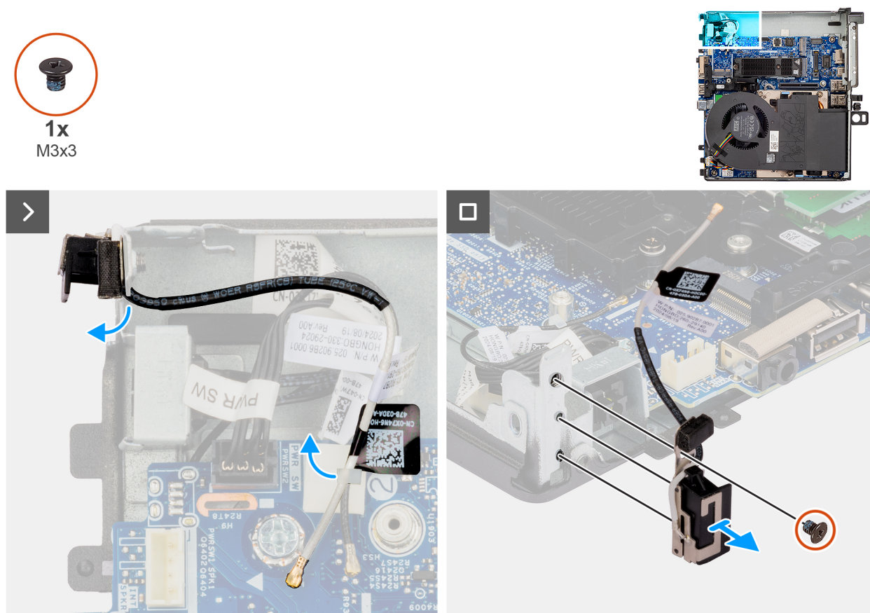
Abbildung 59. Entfernen der internen Antenne – Position 1
