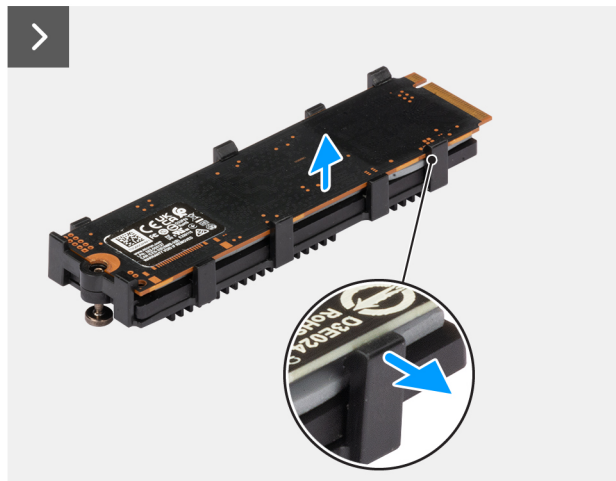
Abbildung 22. Entfernen des M.2-2280-PCIe-Solid-State-Laufwerks (Steckplatz 1)
