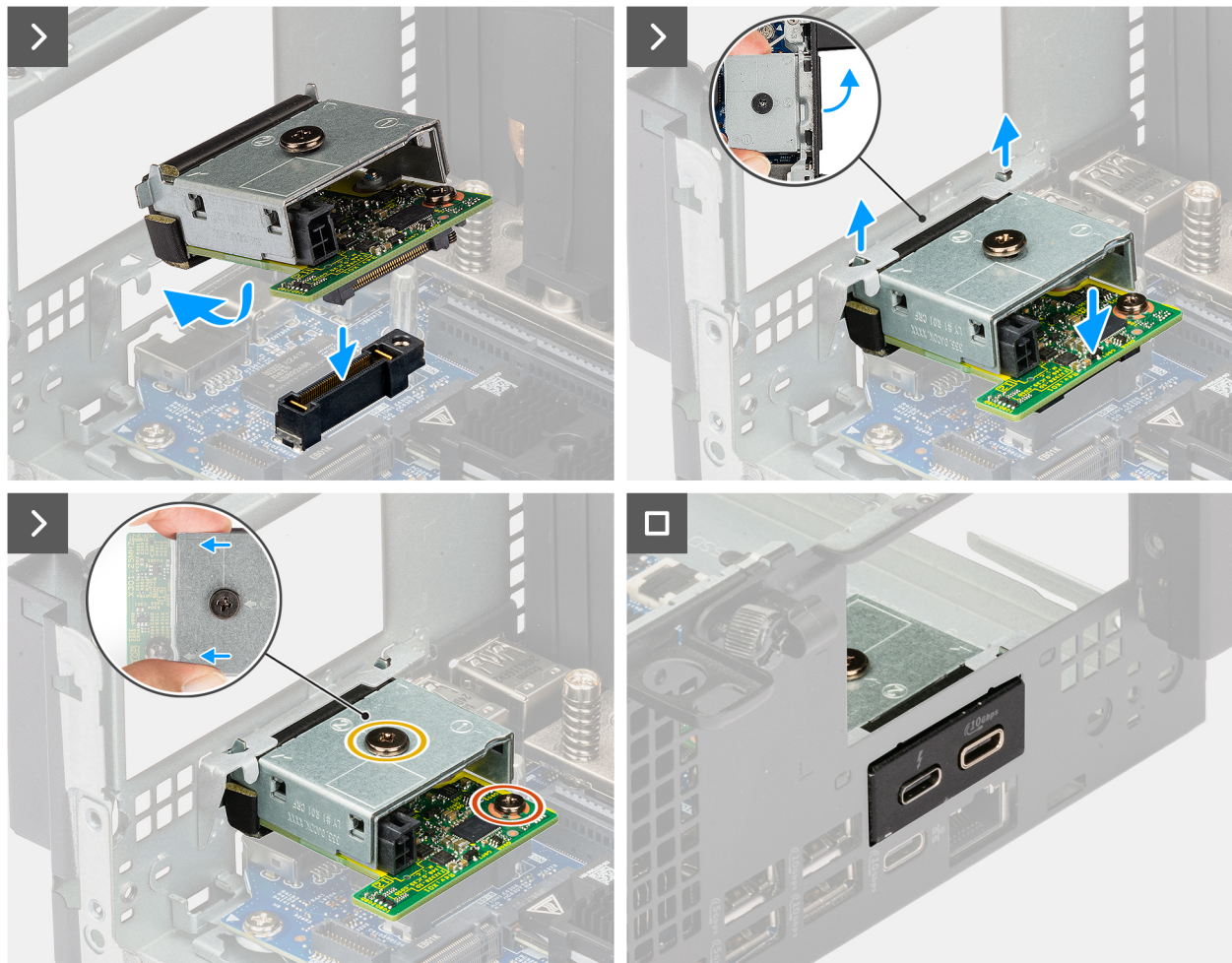
Abbildung 42. Einbauen des Thunderbolt-Anschlusses
