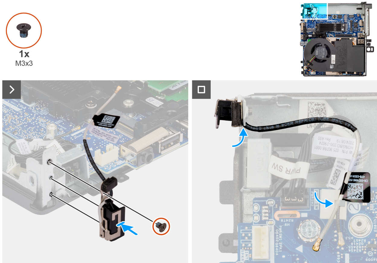
Abbildung 60. Einbauen der internen Antenne – Position 1
