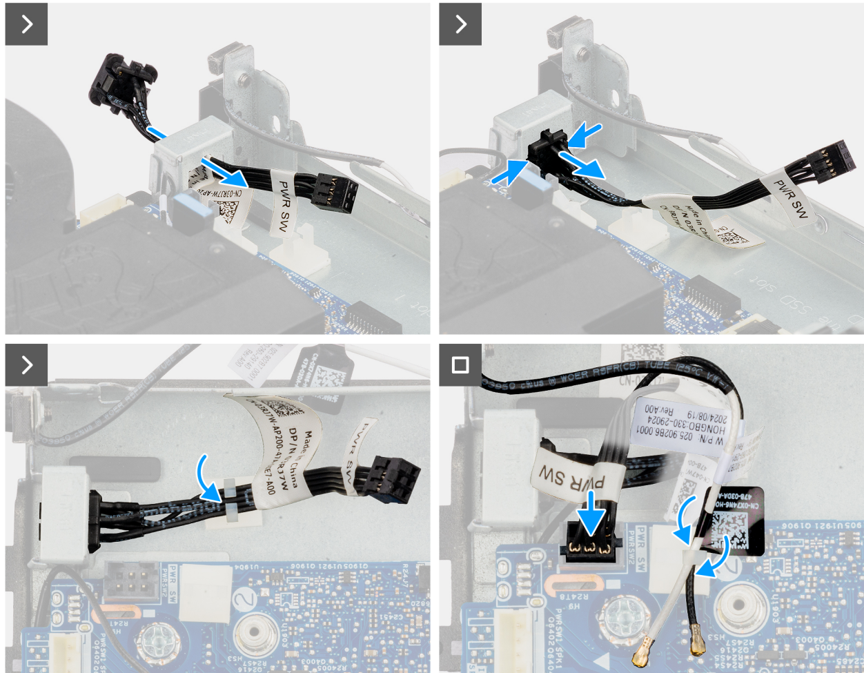
Abbildung 58. Installieren des Netzschalters
