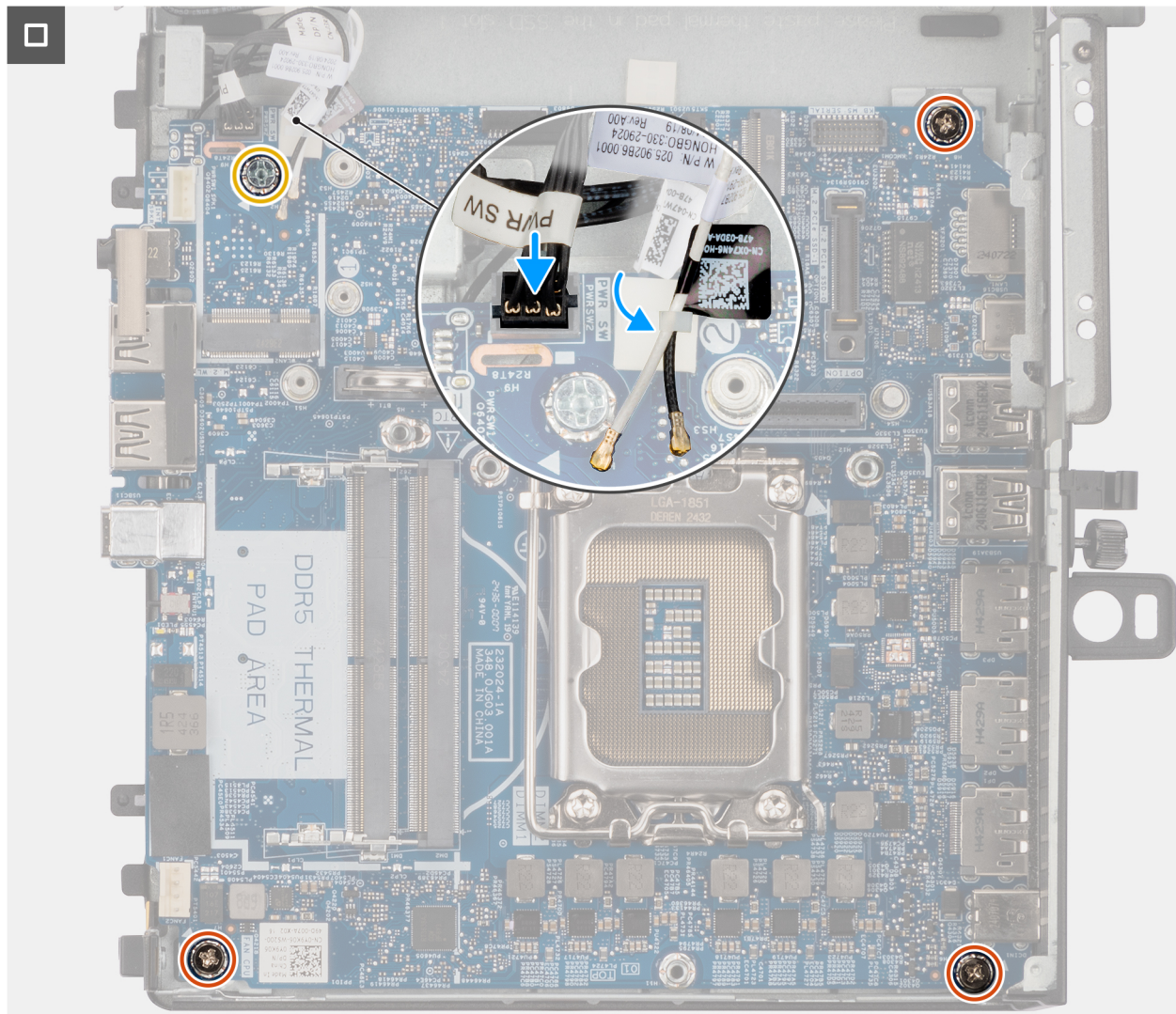
Abbildung 56. Einbauen der Systemplatine
