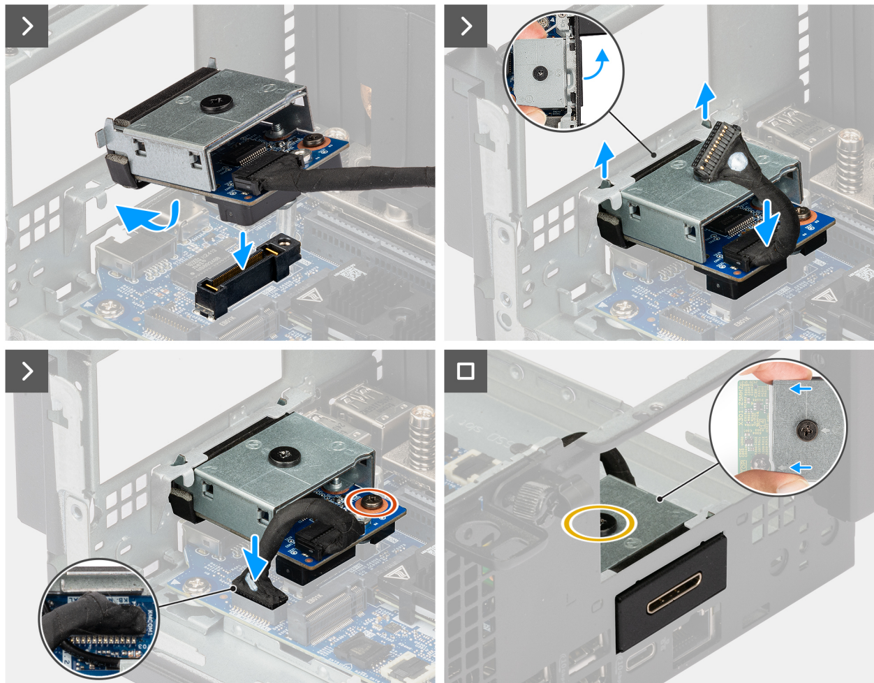
Abbildung 36. Einbauen des PS2-Anschlusses
