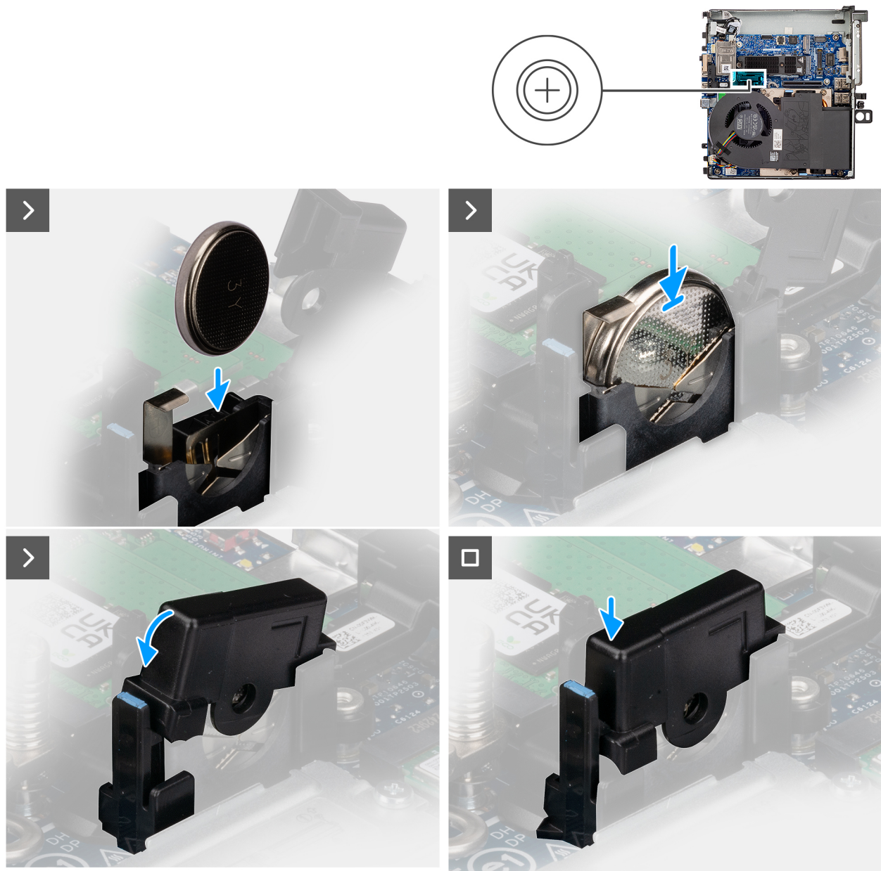
Abbildung 9. Einsetzen der Knopfzellenbatterie
