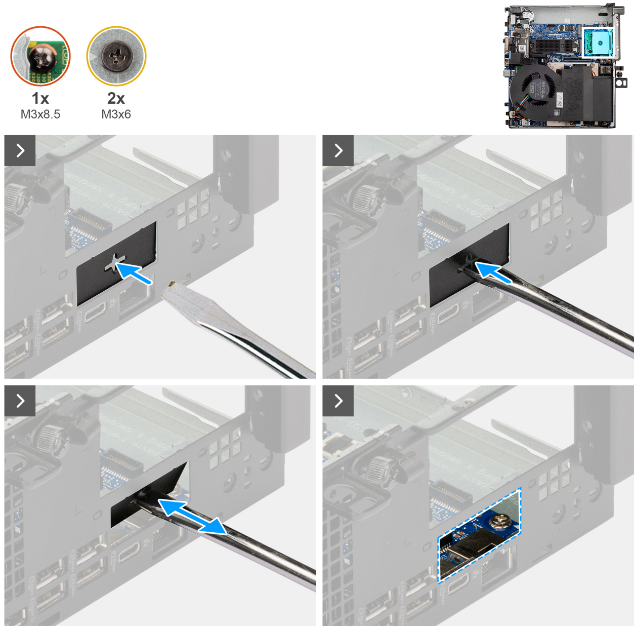
Abbildung 32. Einbauen des optischen 5G-Glasfaseranschlusses
