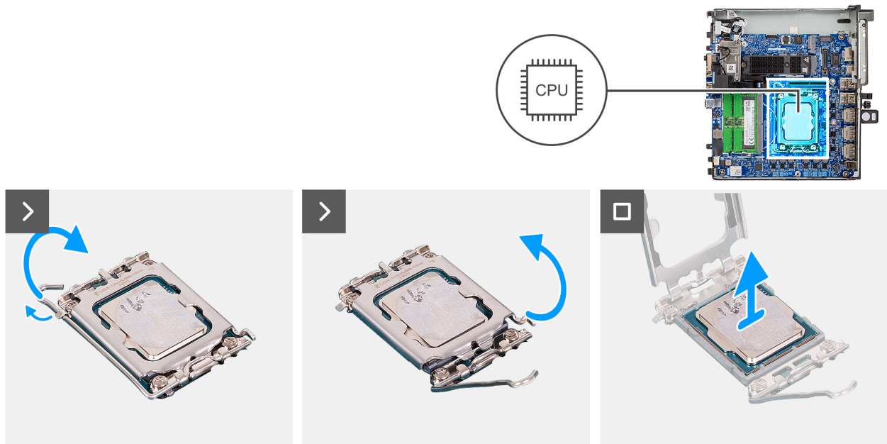
Abbildung 49. Entfernen des Prozessors
