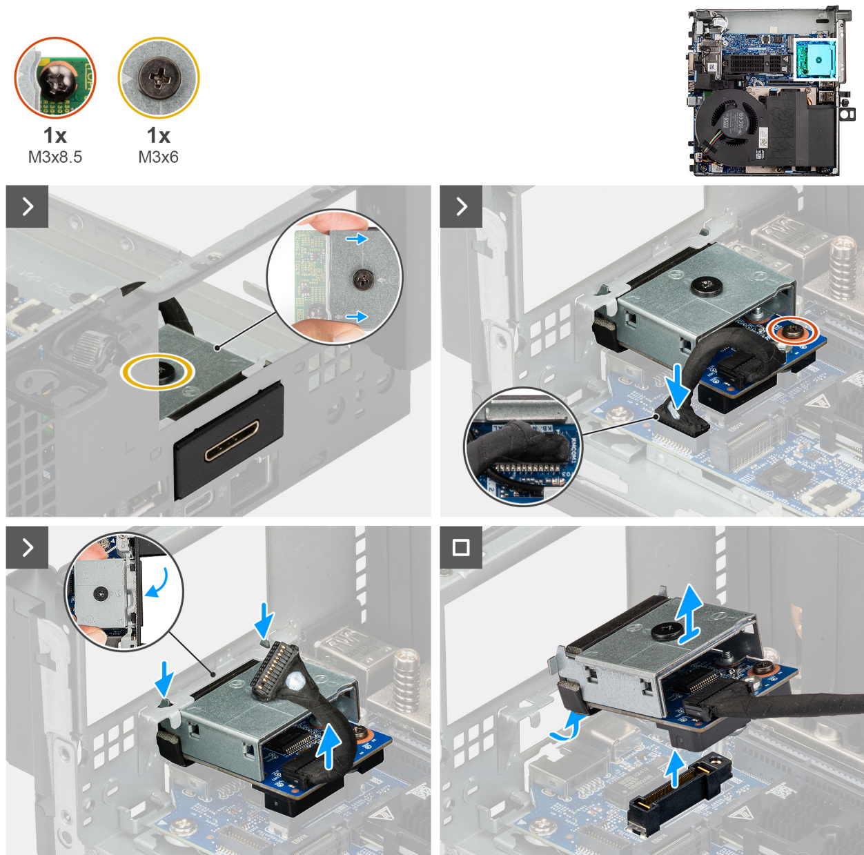
Abbildung 37. Entfernen des PS2-Anschlusses
