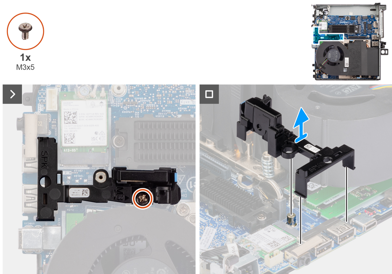
Abbildung 30. Entfernen der Lautsprecherbauhalterung
