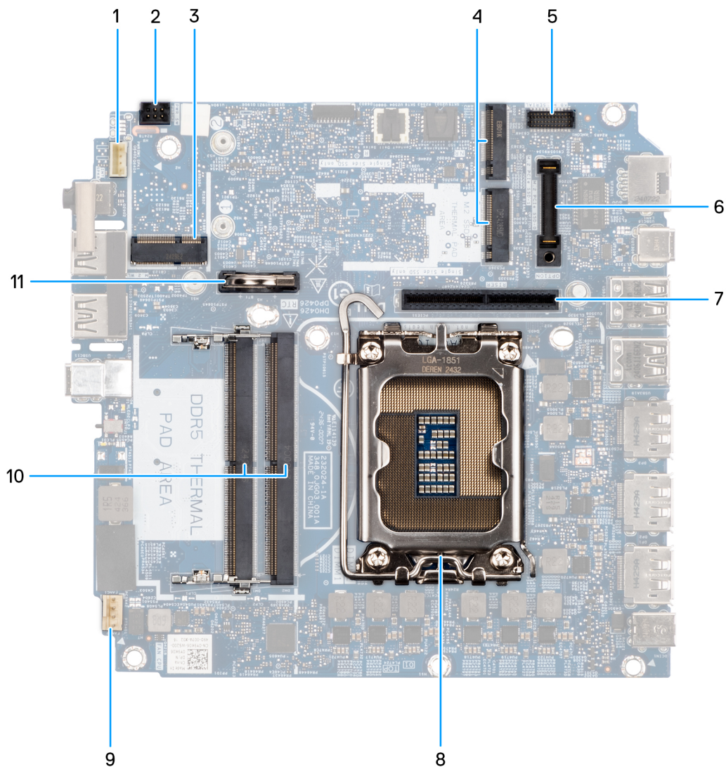
Abbildung 54. Anschlüsse auf der Hauptplatine
