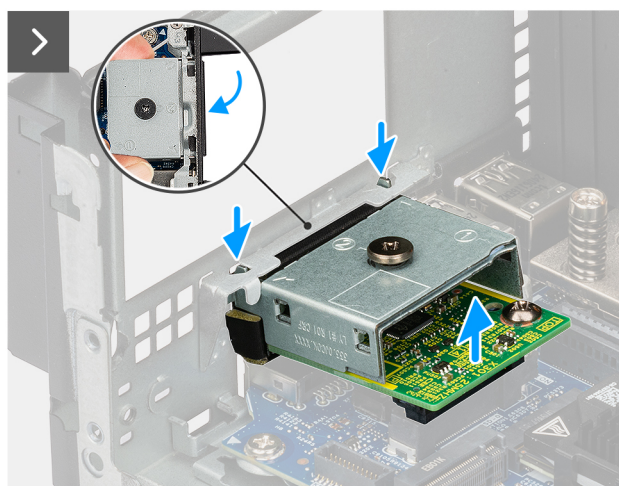
Abbildung 40. Entfernen des DisplayPorts
