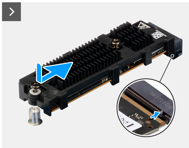
Abbildung 23. Einbauen des M.2-2280-PCIe-SSD-Laufwerks (Steckplatz 1)
