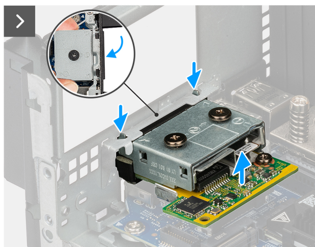
Abbildung 34. Entfernen des optischen 5G-Glasfaseranschlusses
