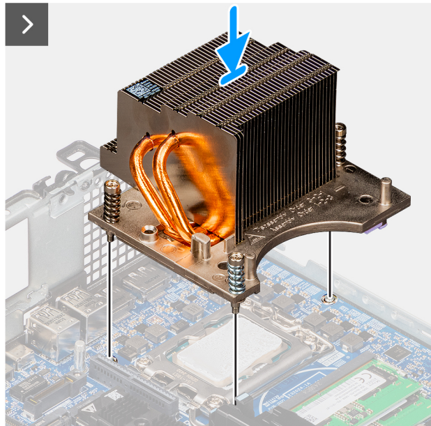
Abbildung 48. Einsetzen des Kühlkörpers
