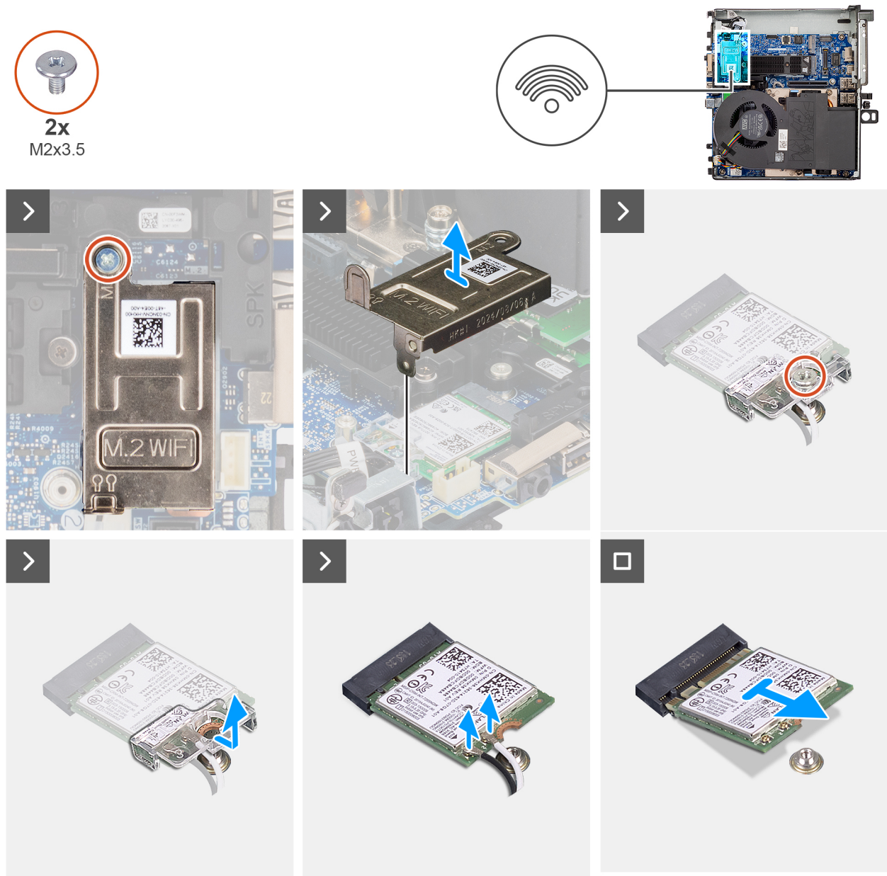
Abbildung 26. Entfernen der Wireless-Karte
