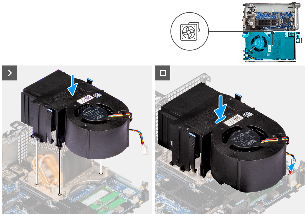
Abbildung 17. Einbauen des Systemlüfters
