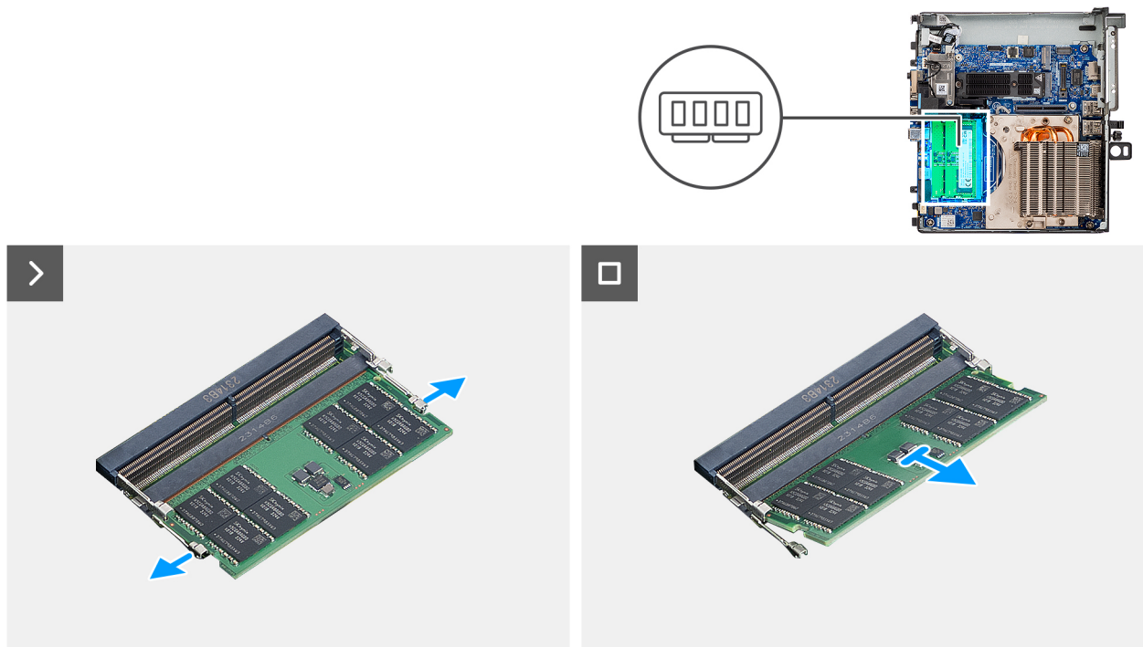
Abbildung 18. Entfernen der Speichermodule
