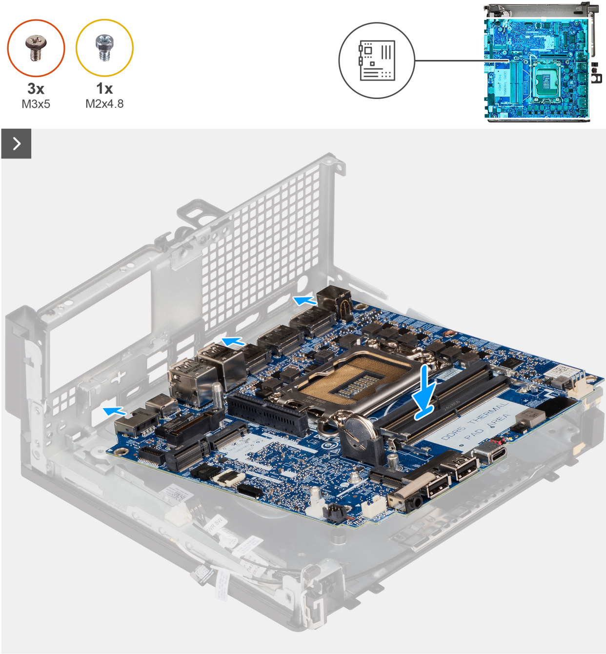
Abbildung 55. Einbauen der Systemplatine
