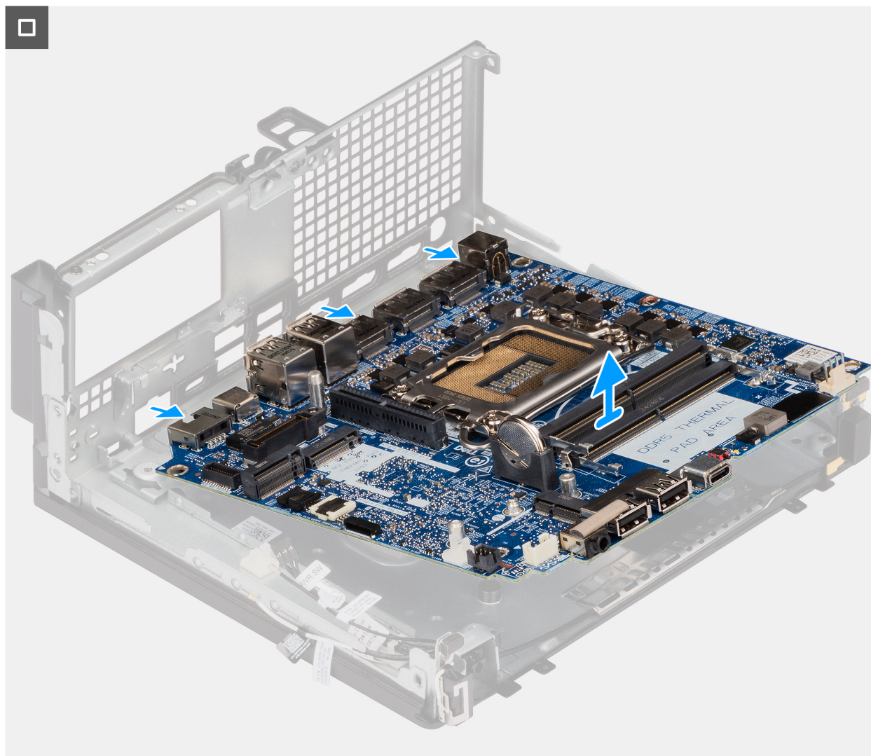
Abbildung 53. Entfernen der Systemplatine
