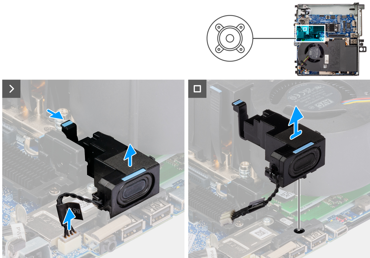
Abbildung 28. Entfernen des Lautsprechers
