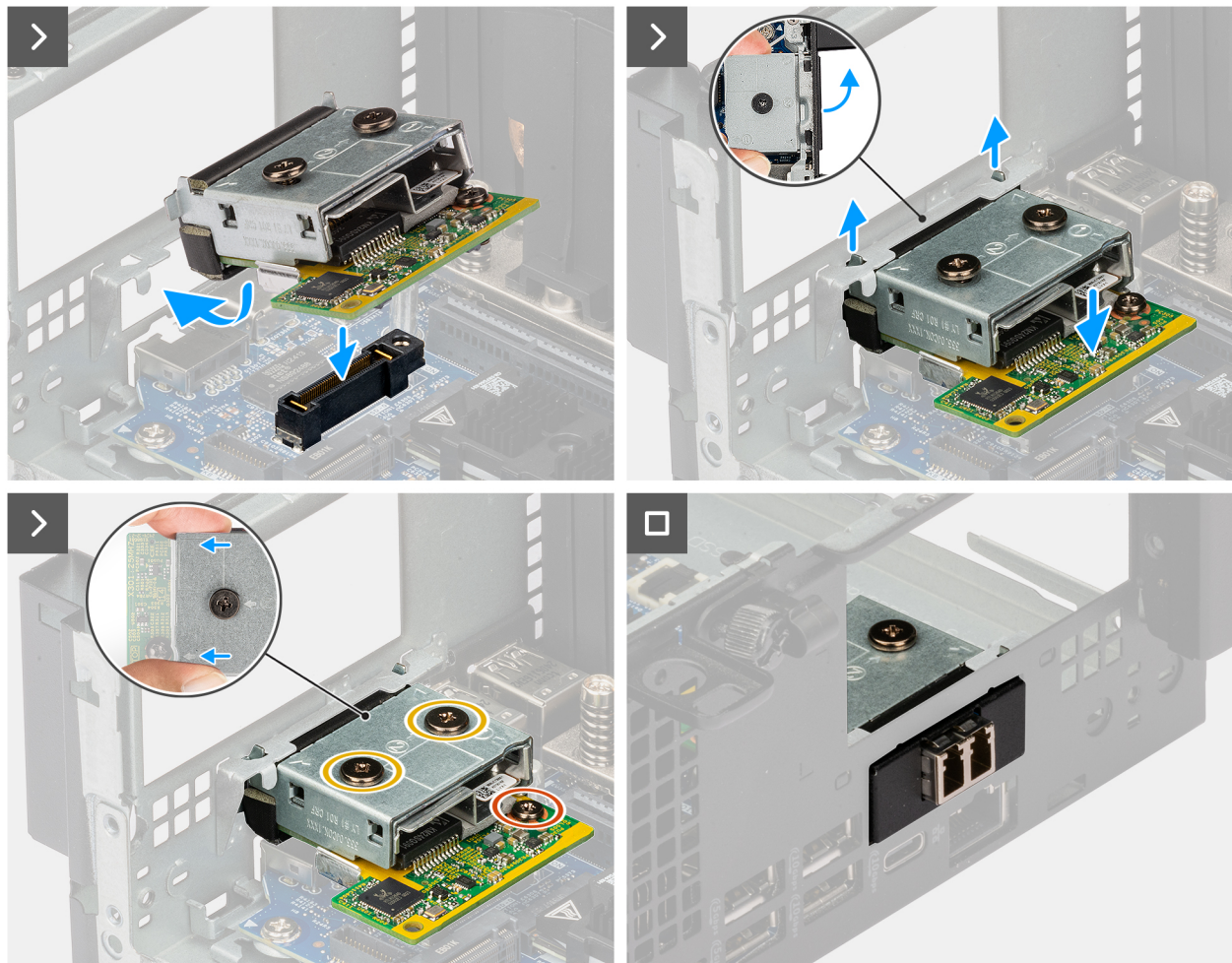
Abbildung 33. Einbauen des optischen 5G-Glasfaseranschlusses
