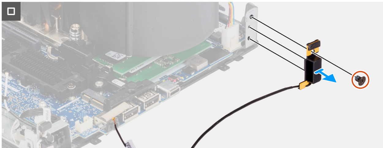
Abbildung 61. Entfernen der internen Antenne – Position 2
