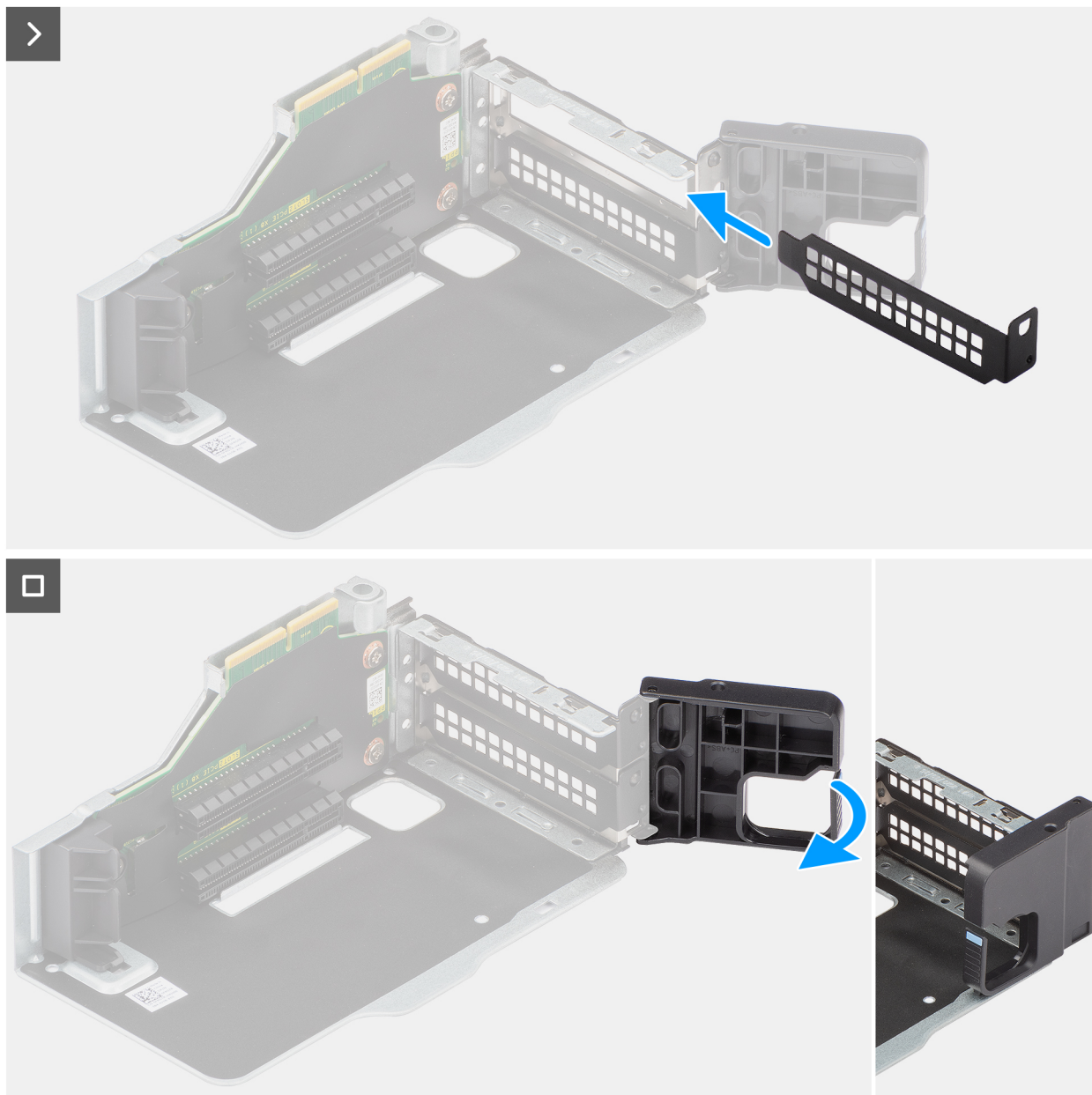
Abbildung 13. Entfernen der Grafikkarte
