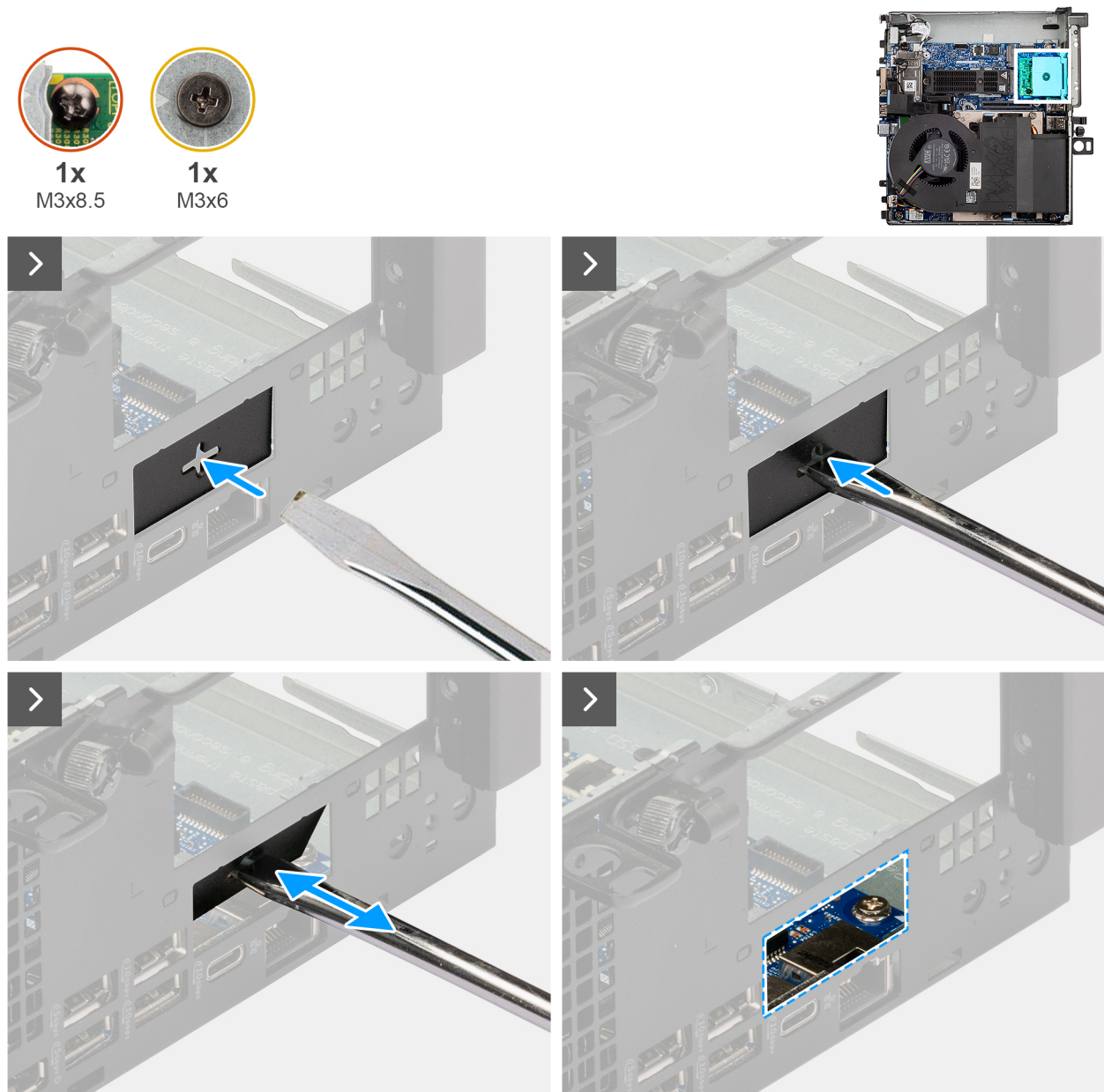
Abbildung 38. Einbauen des DisplayPorts
