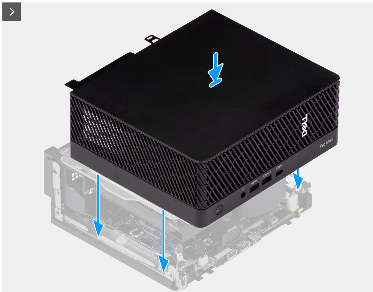
Abbildung 6. Anbringen der Seitenabdeckung
