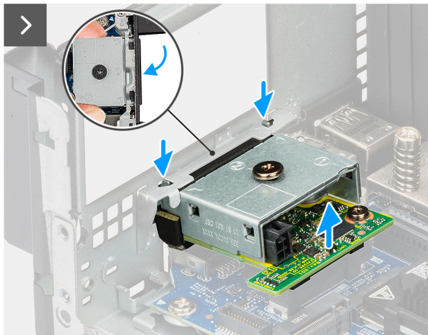
Abbildung 43. Entfernen des Thunderbolt-Anschlusses
