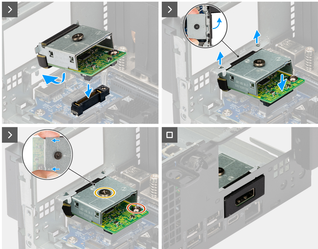
Abbildung 39. Einbauen des DisplayPorts
