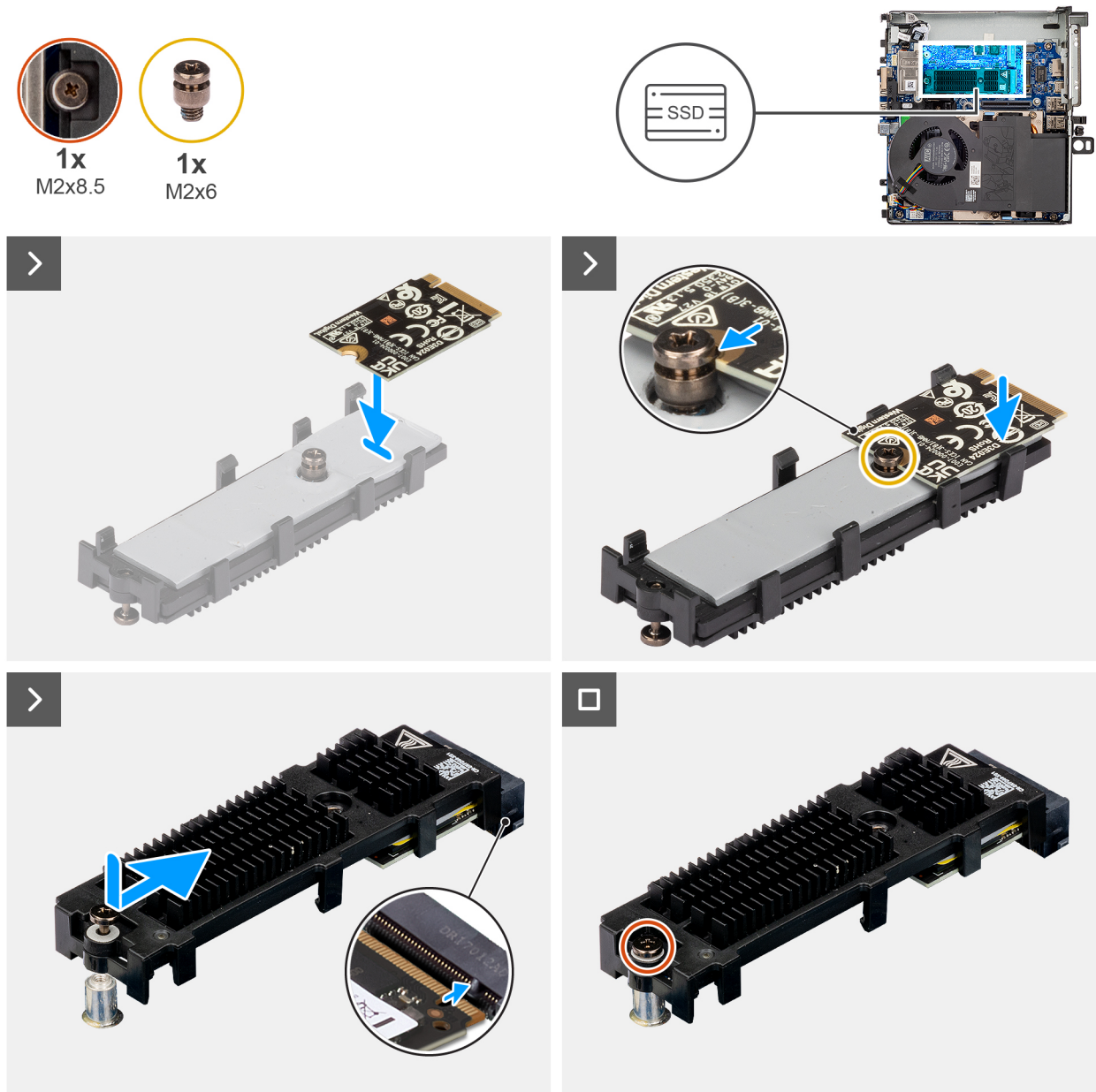
Abbildung 21. Einbauen des M.2-2230-PCle-Solid-State-Laufwerks (Steckplatz 1)
