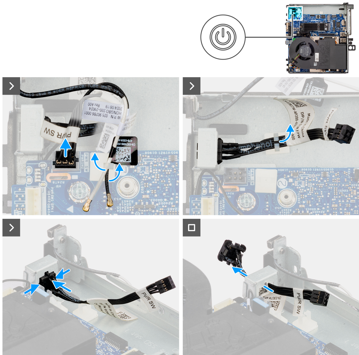
Abbildung 57. Entfernen des Netzschalters
