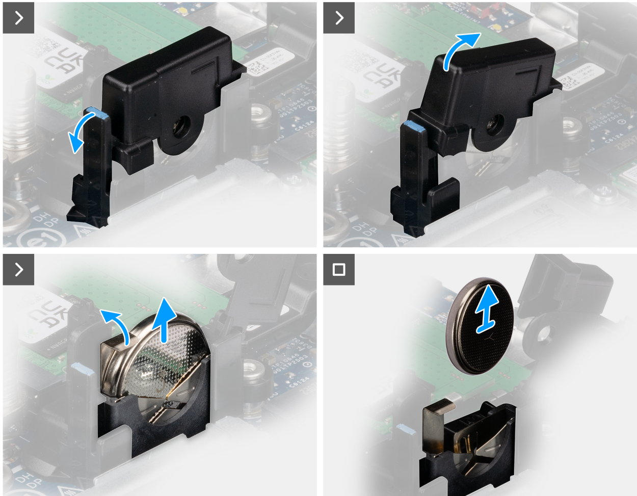
Abbildung 8. Entfernen der Knopfzellenbatterie
