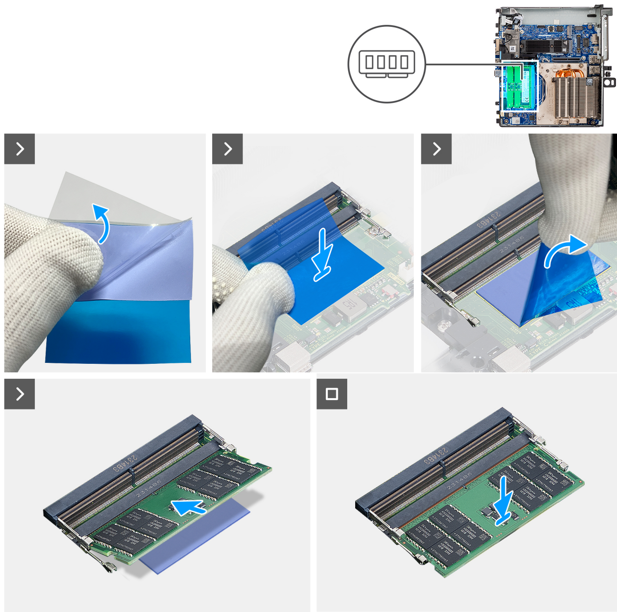
Abbildung 19. Installieren der Speichermodule
