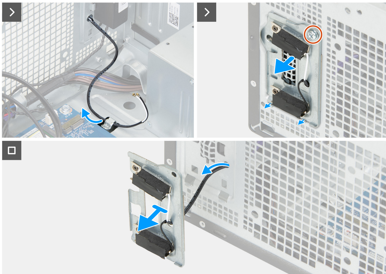
Abbildung 86. Entfernen der Antennenmodule
