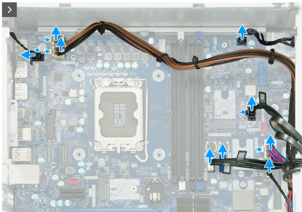
Abbildung 98. Entfernen der Systemplatine
