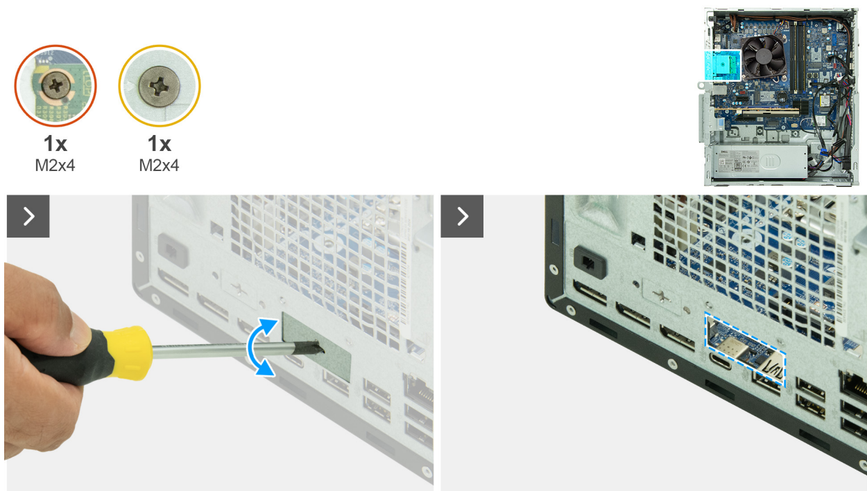
Abbildung 76. Installieren des optionalen Portmoduls
