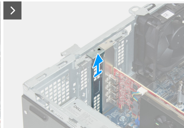
Abbildung 48. Installieren der Halterung der Solid-State-Laufwerk-Erweiterungskarte
