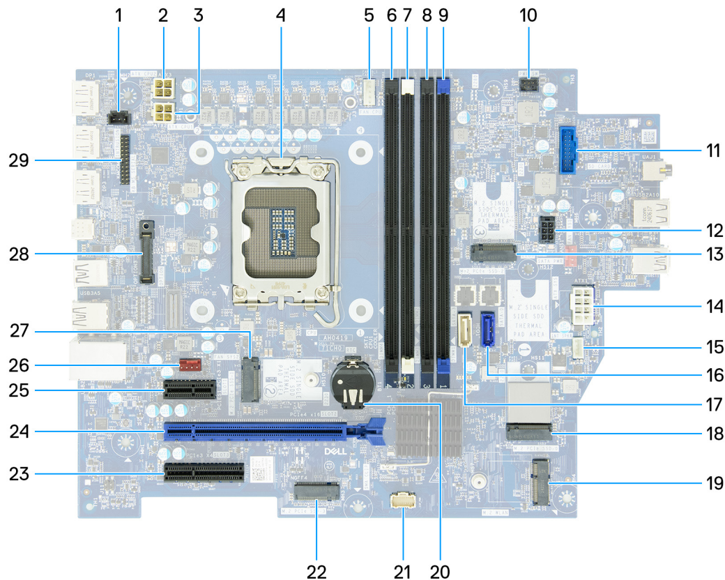
Abbildung 101. Systemplatinenbeschriftung
