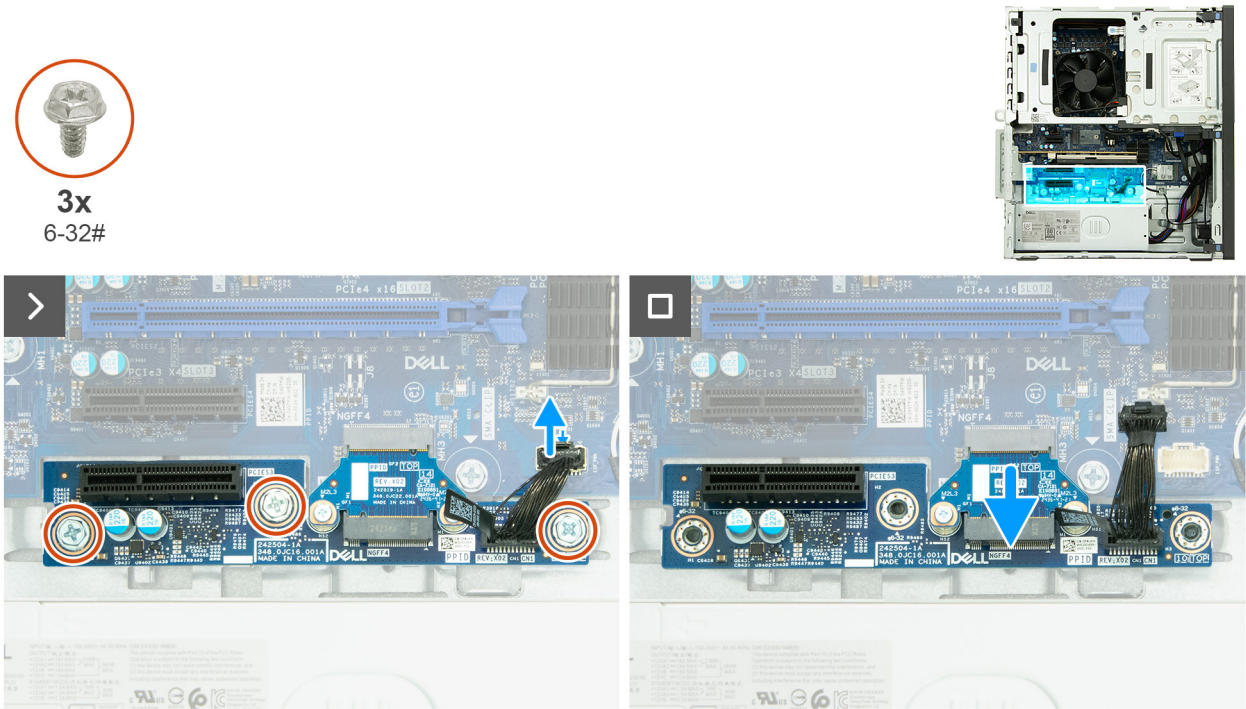
Abbildung 44. Entfernen der PCIe-Erweiterungsplatine
