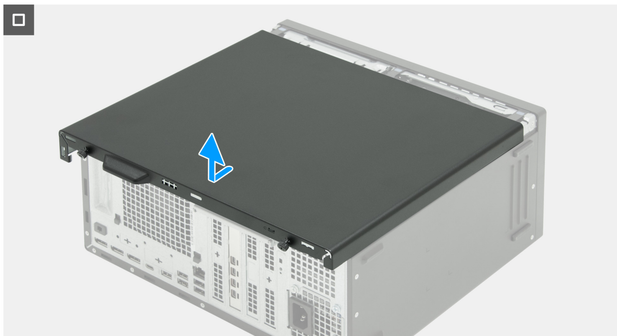
Abbildung 14. Entfernen der linken Abdeckung
