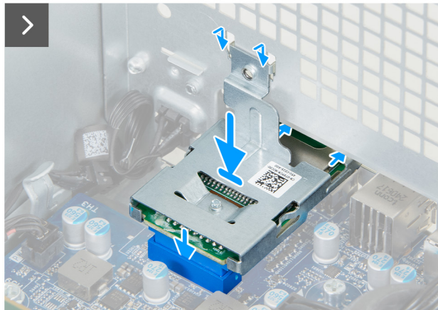
Abbildung 85. Einbauen des Medienkartenlesers
