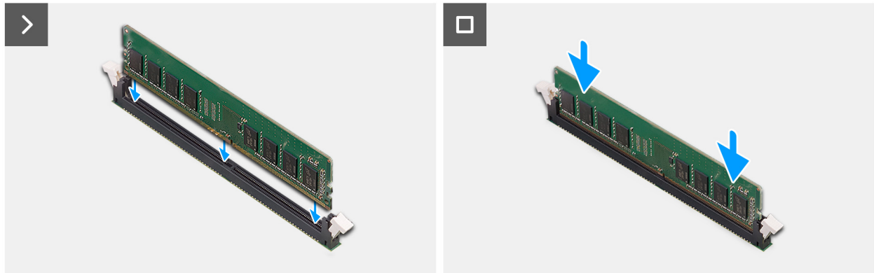
Abbildung 28. Einbauen des Speichers
