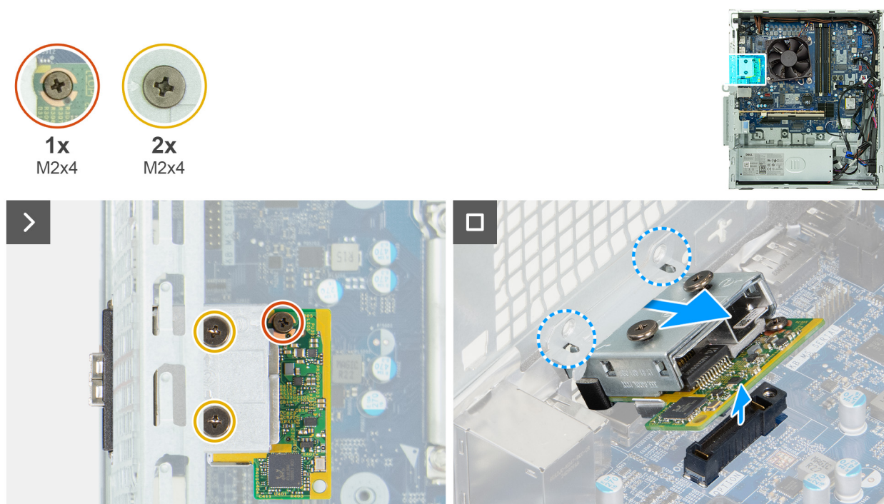
Abbildung 78. Entfernen des Faseroptik-Portmoduls
