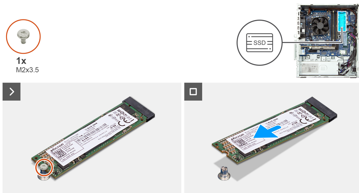
Abbildung 38. Entfernen des M.2 2280-SSD-Laufwerks aus Steckplatz 2
