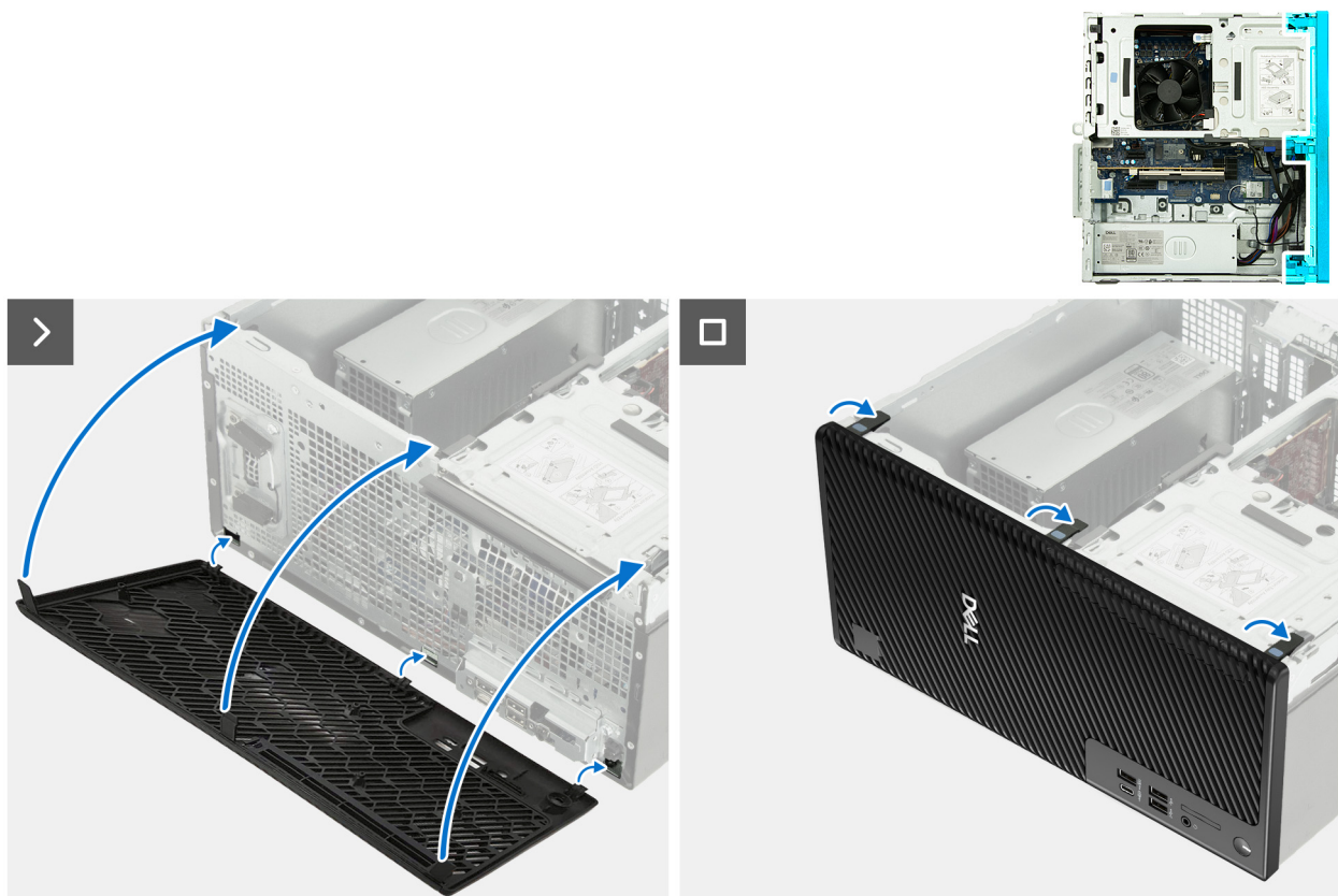
Abbildung 24. Installieren der vorderen Abdeckung
