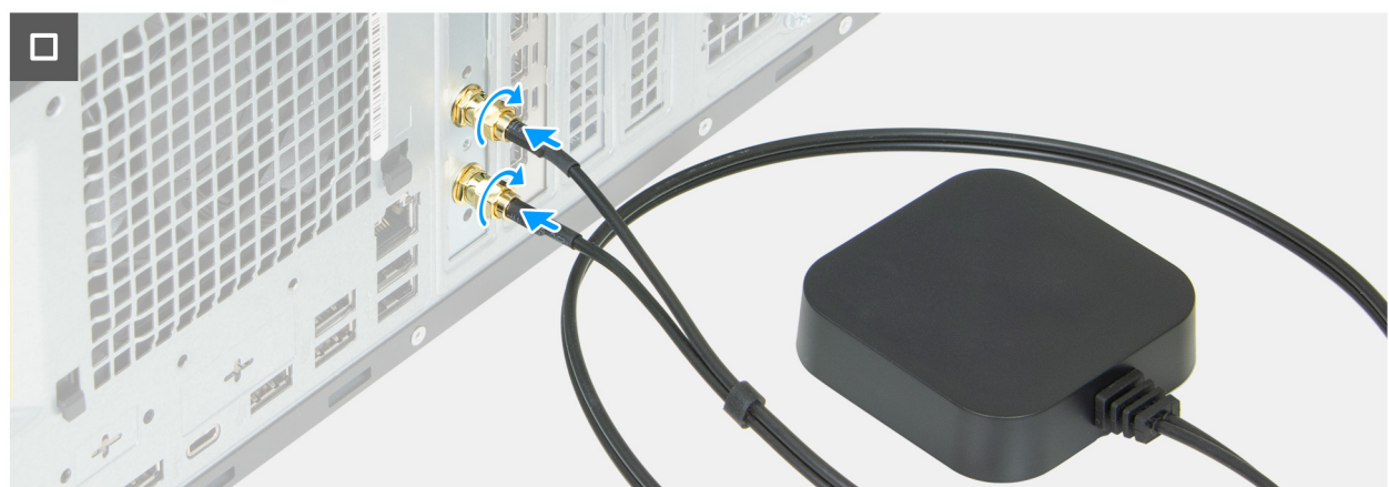
Abbildung 53. Installieren der Puck-Antennen-Erweiterungskarte
