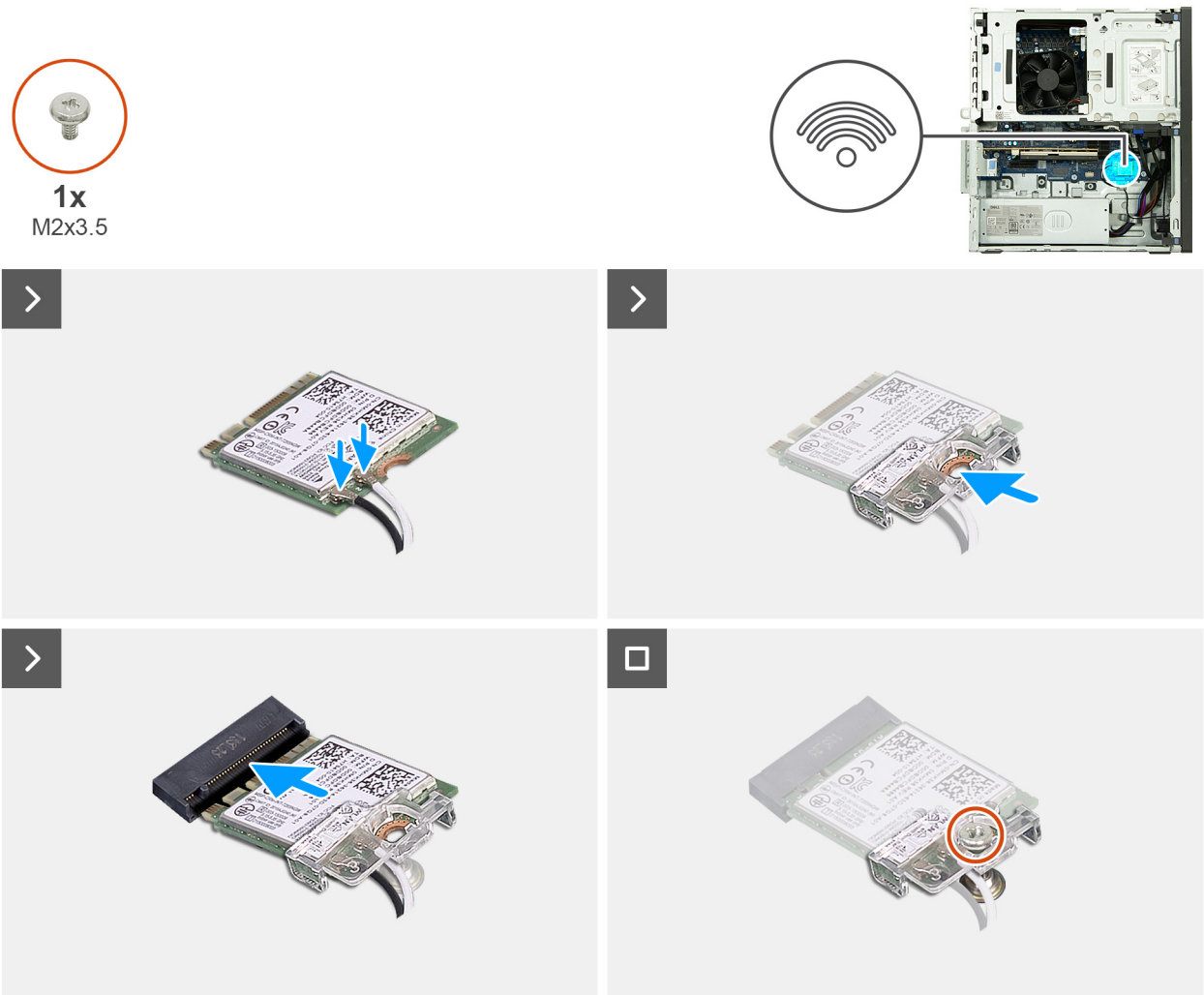
Abbildung 43. Installieren der Wireless-Karte
