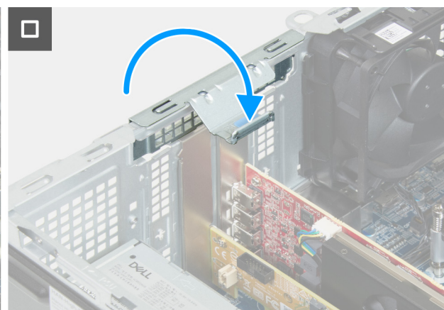
Abbildung 49. Installieren der Halterung der Solid-State-Laufwerk-Erweiterungskarte
