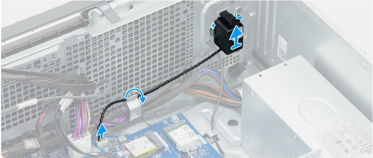
Abbildung 25. Entfernen des internen Lautsprechers
