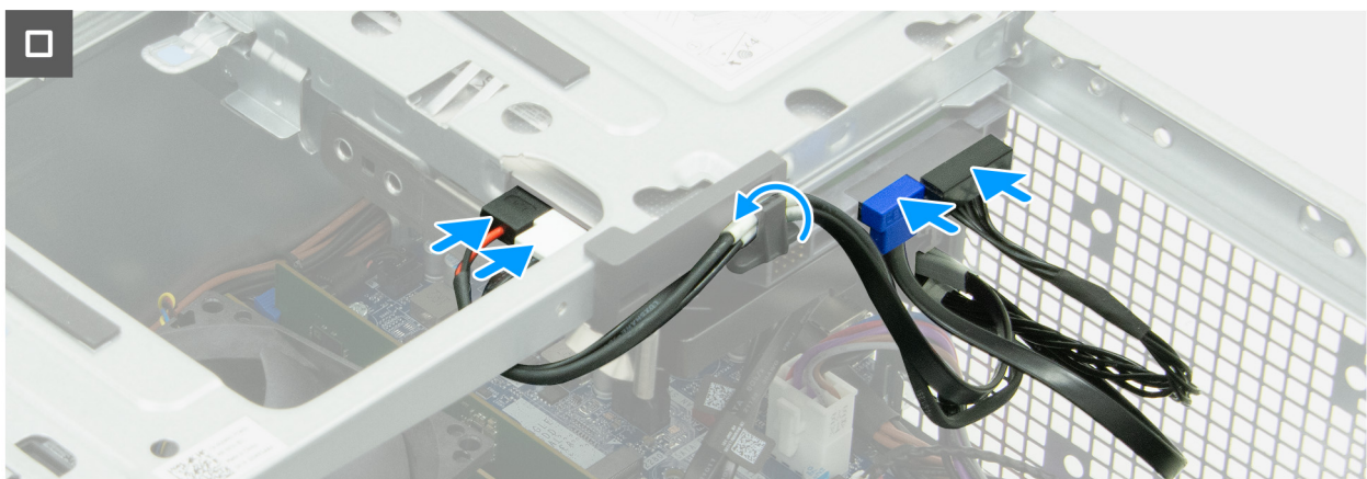
Abbildung 62. Einbauen des Laufwerkschachts
