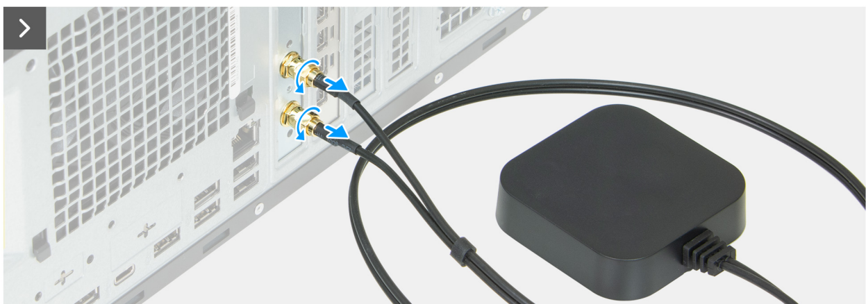
Abbildung 50. Entfernen der Puck-Antennen-Erweiterungskarte
