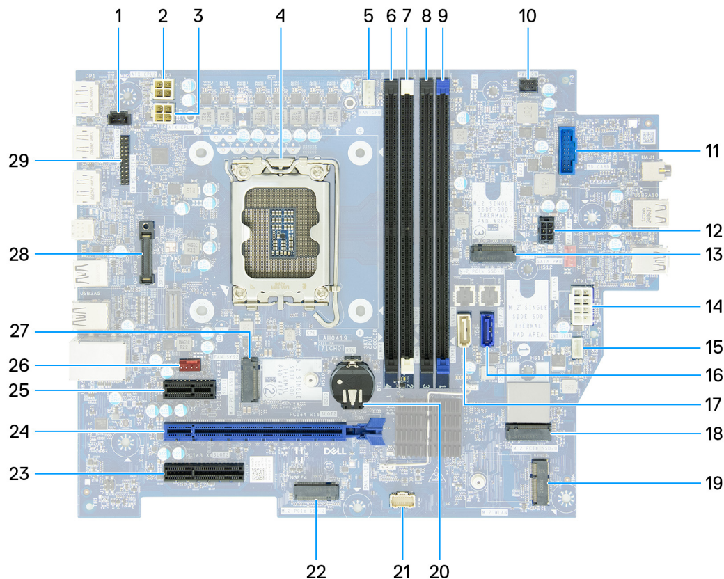
Abbildung 96. Systemplatinenbeschriftung
