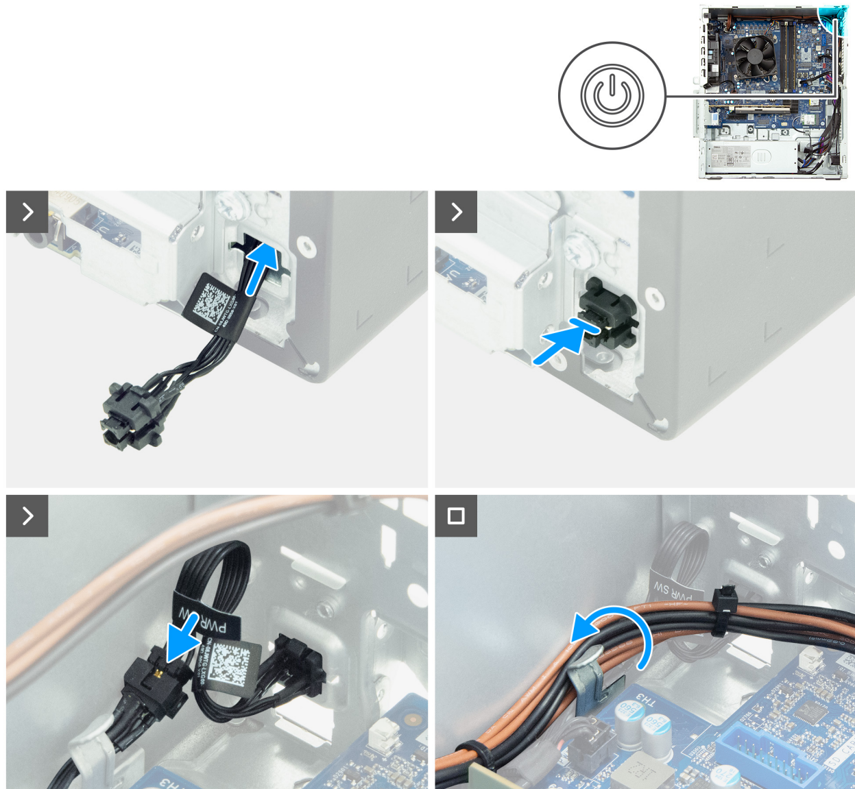
Abbildung 74. Installieren des Netzschalters
