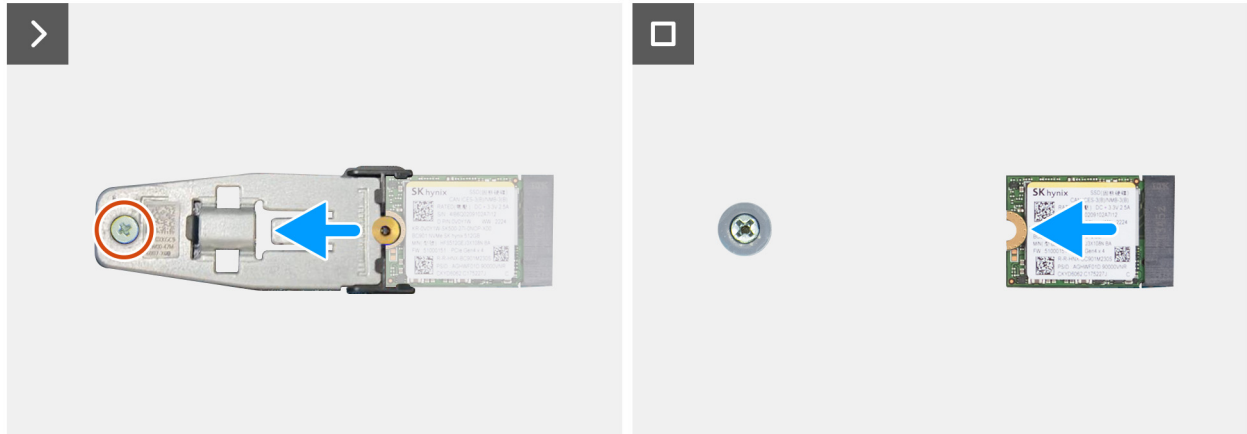
Abbildung 36. Entfernen des M.2 2230-SSD-Laufwerks aus Steckplatz 2
