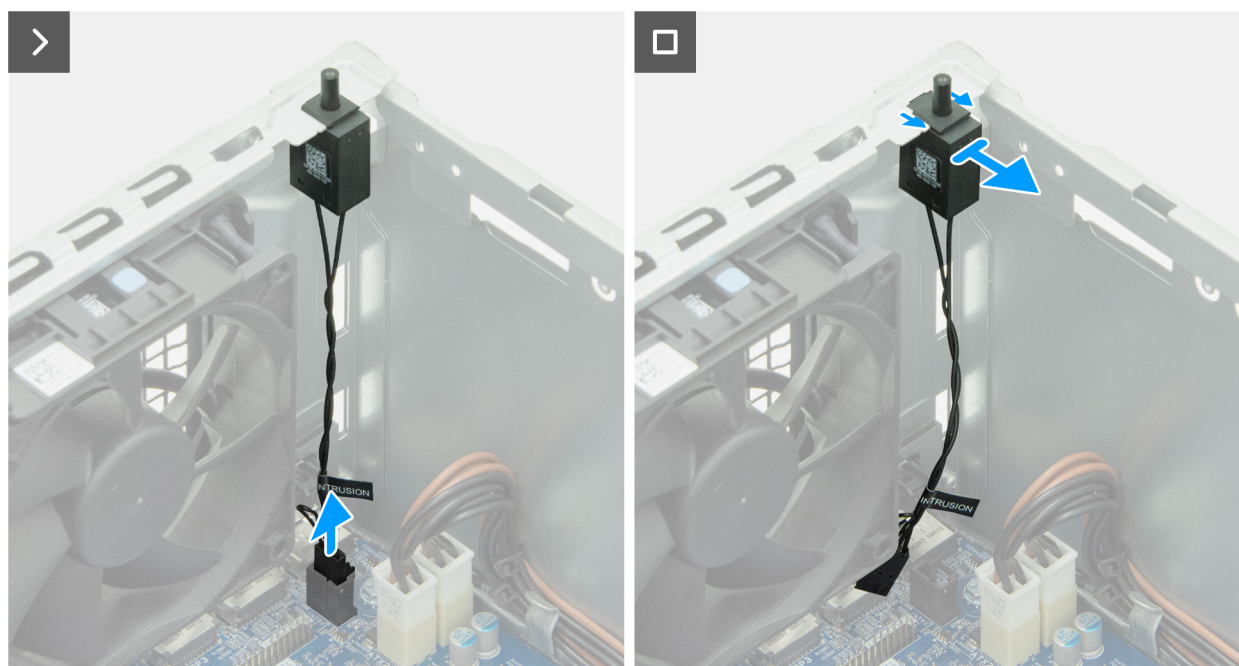
Abbildung 65. Entfernen des Eingriffsschalters
