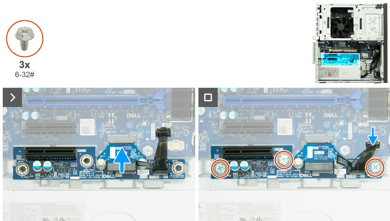
Abbildung 45. Einbauen der PCIe-Erweiterungsplatine
