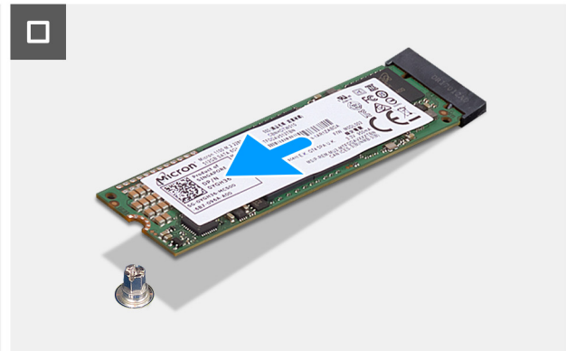
Abbildung 31. Entfernen des M.2 2280-Solid-State-Laufwerks aus Steckplatz 0
