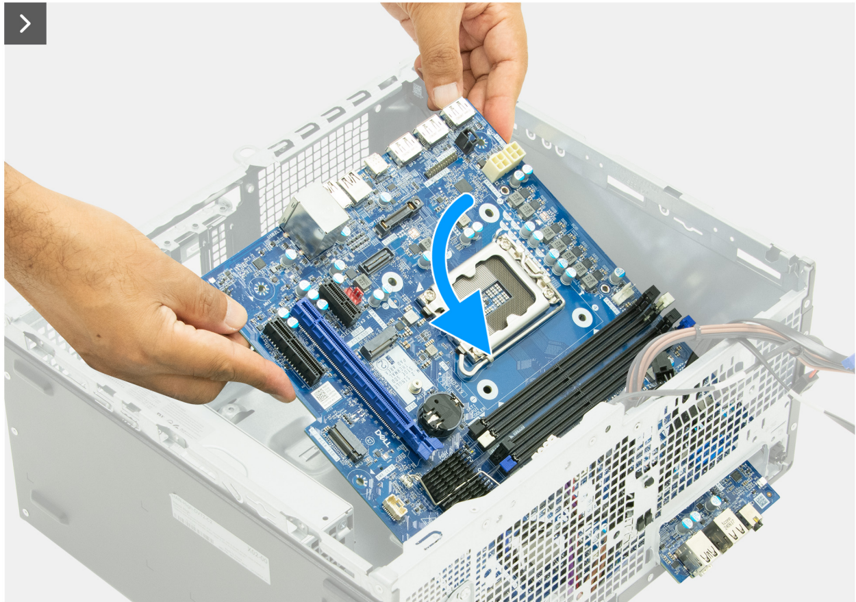
Abbildung 102. Einbauen der Systemplatine
