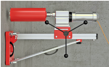
Diamantbohrgeräte
