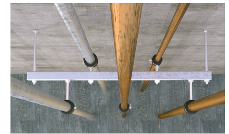
Abgehängte Montageschienen
