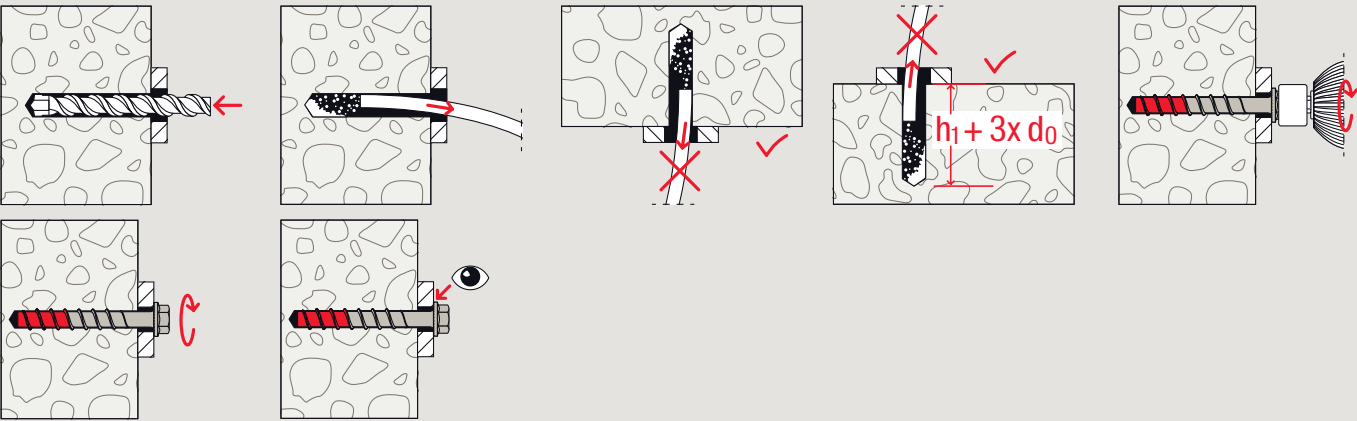
Justage Anbauteil
