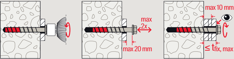
Justage Anbauteil
