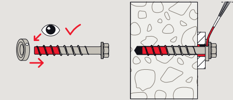
Ringspaltverfüllung
