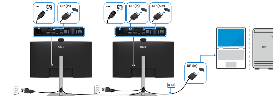
Abbildung 32. Anschließen des Monitors für die DisplayPort Multi-Stream Transport (MST)-Funktion
