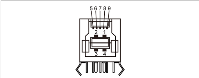
Abbildung 10. USB Type-B 5 Gbit/s Upstream-Anschluss
