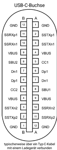
Abbildung 9. USB-C-Anschluss
