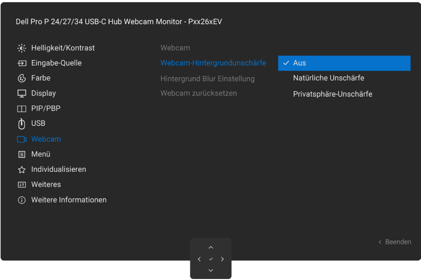
Abbildung 5. Webcam-Hintergrundunschärfe
