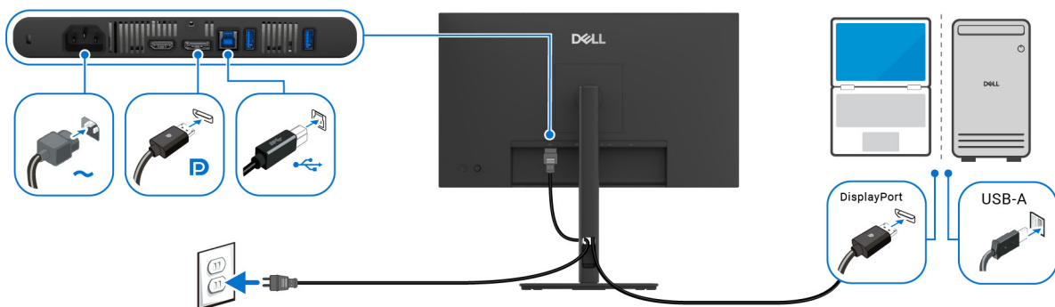
Abbildung 30. DisplayPort Verbindung
