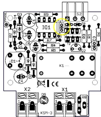
Bestückungsplan Hardware-Version 2
