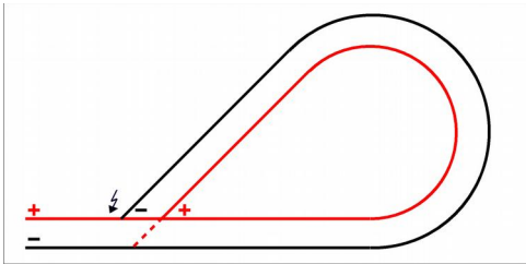
Abbildung: Kurzschluss-Problematik an der Weiche einer Kehrschleife
