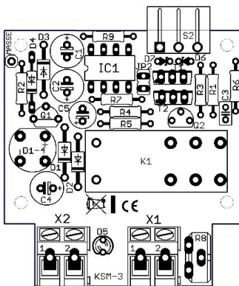
Bestückungsplan Hardware-Version 1
