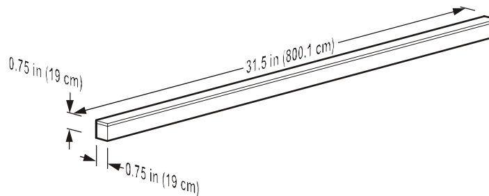
Abdämmungsstreifen (4)
