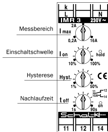
IMR 3 Bedienelemente
